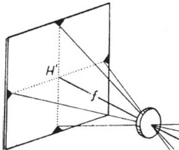
Obrázek 5: Vnitřní orientace snímku [3]
