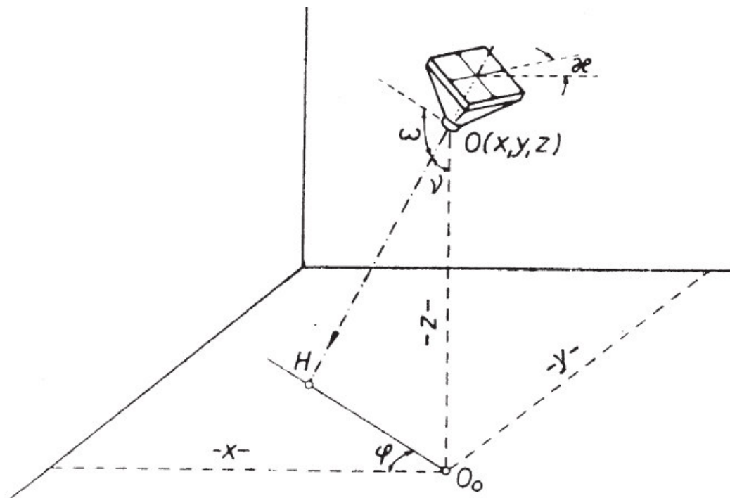
Obrázek 6: Prvky vnější orientace snímku [3]
