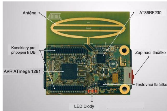
Obrázek 4.1: Popis modulu s rádiem (RCB) [6]
