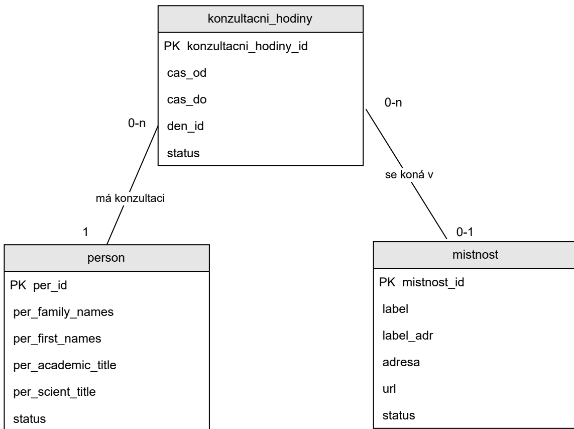
Obrázek C.2: ER diagram popisující konání konzultačních hodin vyučujících
