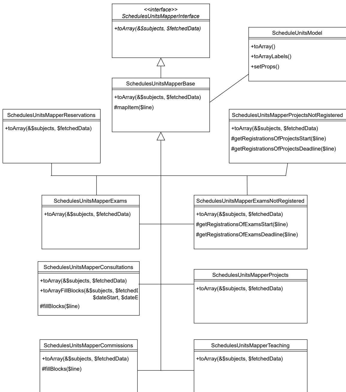
Obrázek B.2: Diagram tříd znázorňující navrženou architekturu mapování dat z databáze na modely
