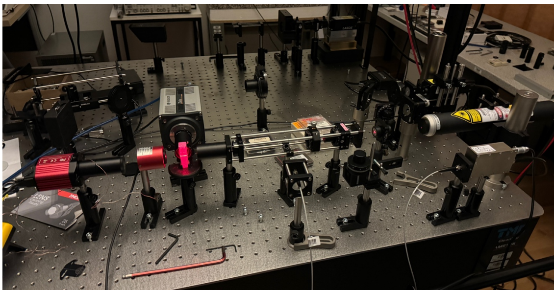
Obrázek 7.1: Sestavená aparatura
