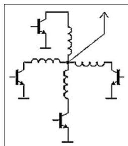
Obr. 1.7: Principiální schéma unipolárního zapojení, převzato z [2]
