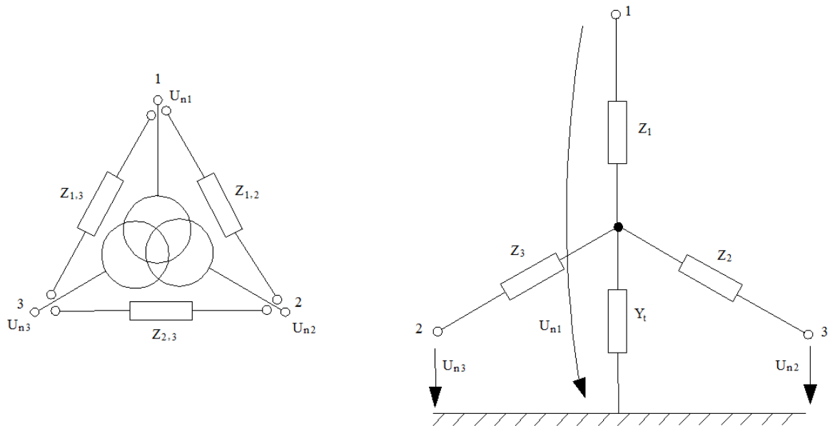
Obr. 1-3 Náhradná schéma trojvinuťového transformátora
