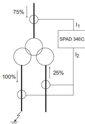
Obr. 8-7 Zapojenie ochrany na trojvinuťový transformátor
