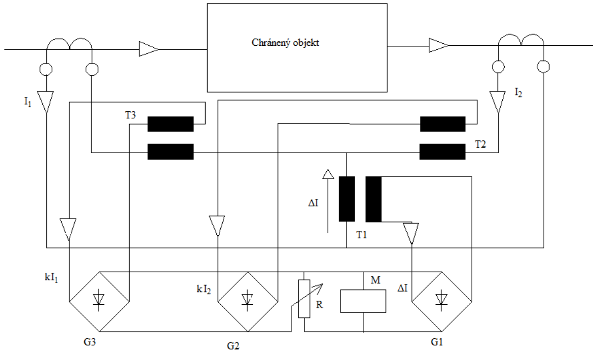
Obr. 5-7 Spôsob kompenzácie pomocou rozdielového členu s usmerňovačmi
