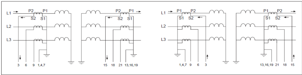
Obr. 8-4 Typové zapojenie prúdových transformátorov - typ II
