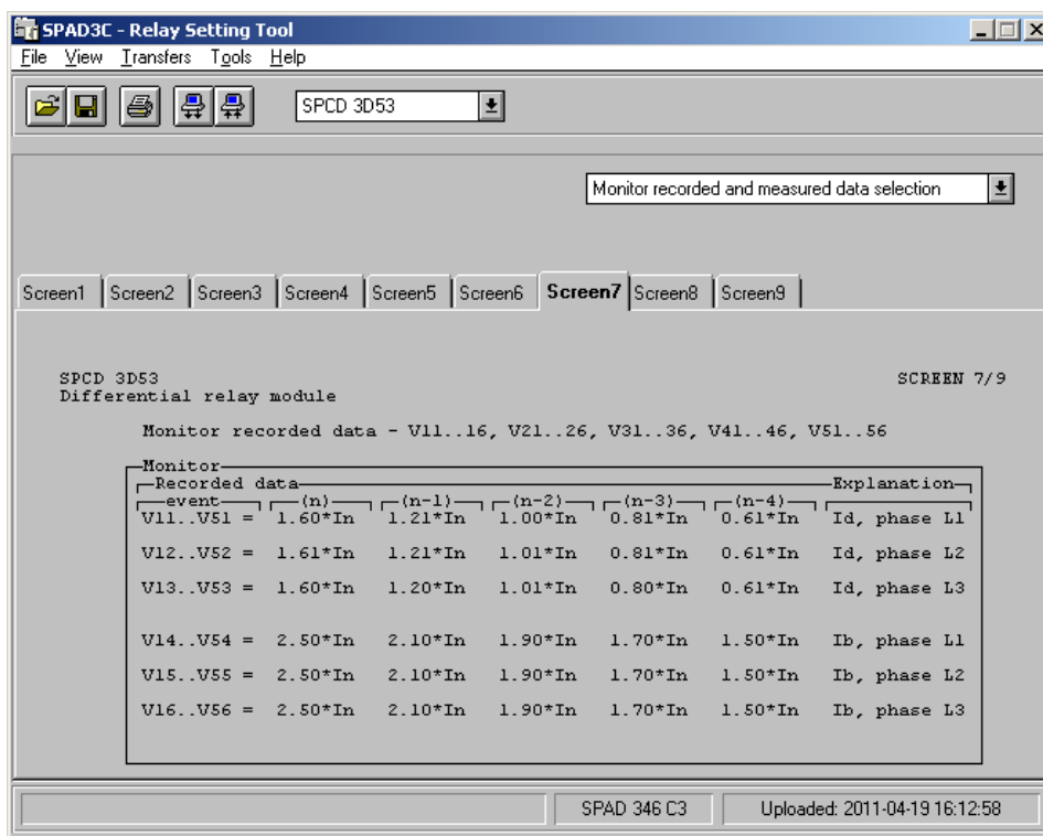
Obr.11-2 Hodnoty diferenciálneho a stabilizačného prúdu ochrany
