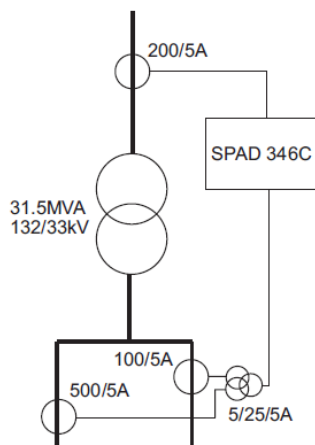
Obr. 8-6 Zapojenie ochrany na dvojvinuťový transformátor s dvoma výstupmi
