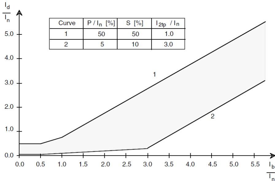
Obr. 8-2 Medzné vypínacie charakteristiky
