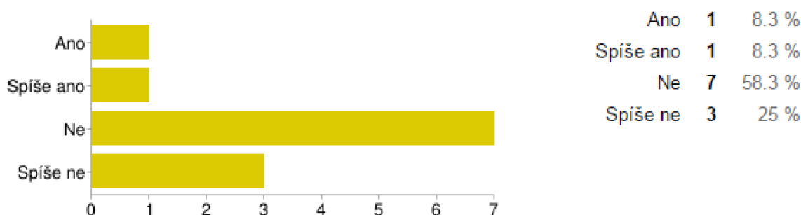
Graf č. 6 - Schopnost hradit finanční ztrátu (Vlastní zpracování)
