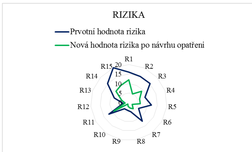
Graf č. 10 - Pavučinový graf (Vlastní zpracování)
