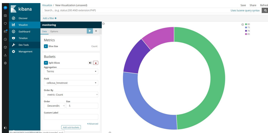
Obr. 3.1: Kibana.
