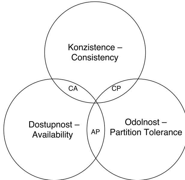
Obr. 2.1: CAP teorém.
