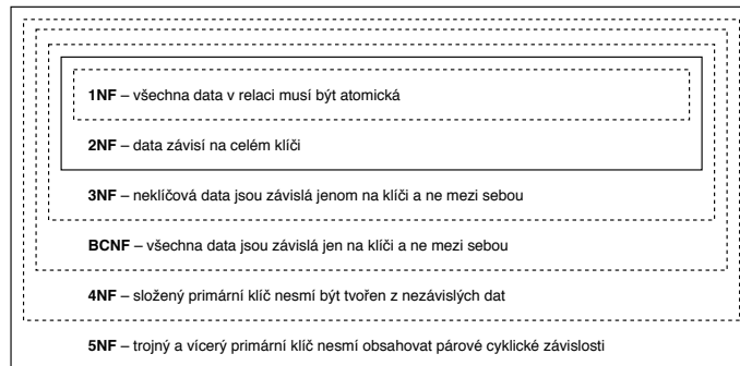
Obr. 1.1: Normální formy.
