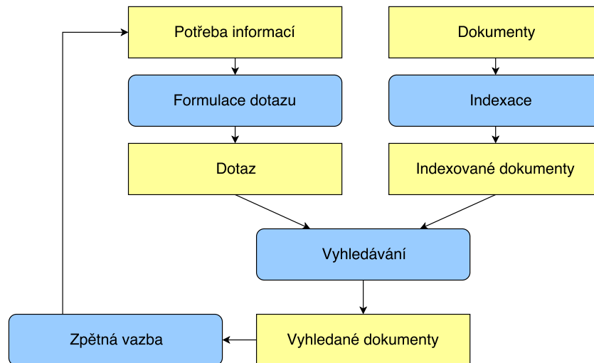
Obr. 3.2: Fulltextové vyhledávání.
