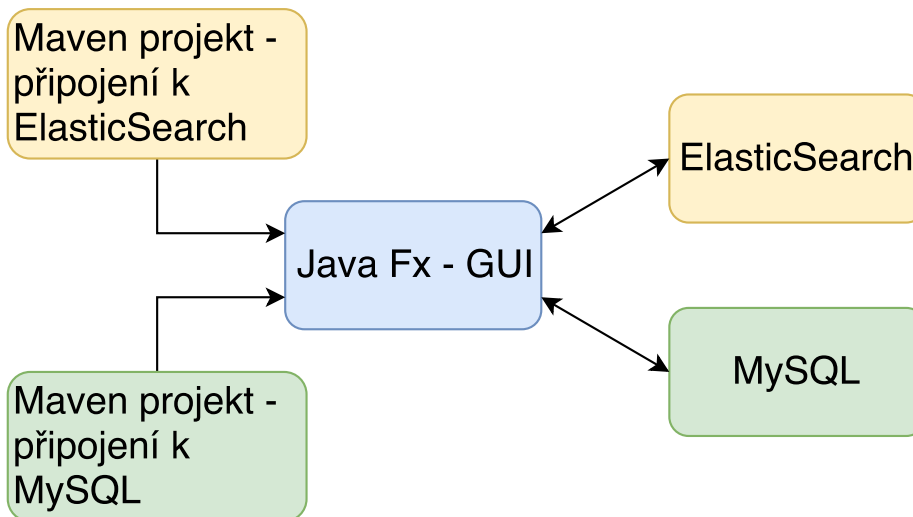
Obr. 4.3: Schéma aplikace.
