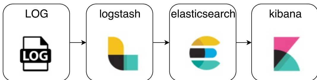
Obr. 3.3: Schéma logování.
