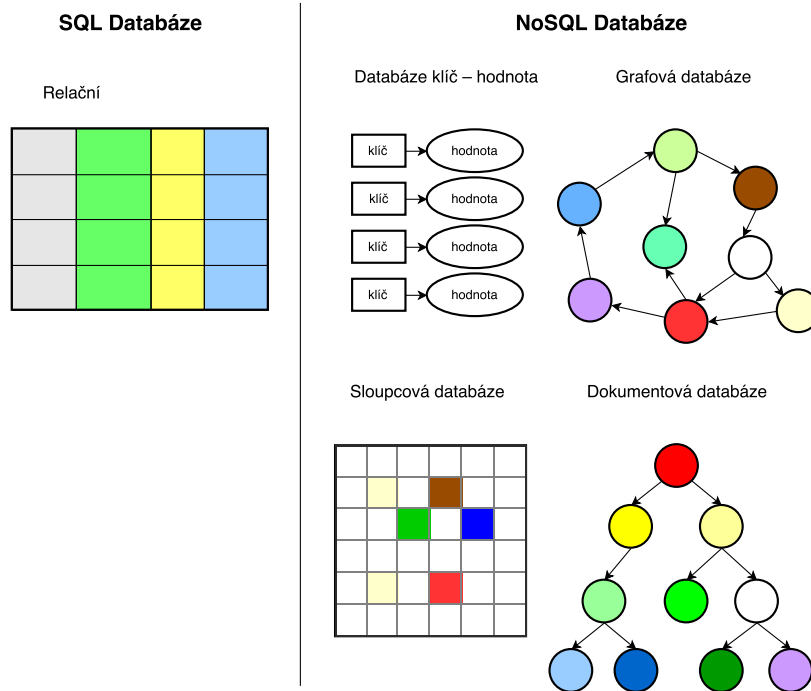
Obr. 2.2: Srovnání databází.
