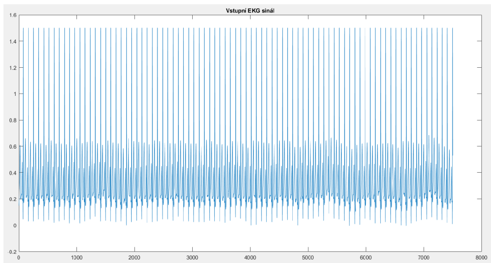
Obr. 3.6: Ukázka vstupního EKG signálu (signál č. 42 1000-8500 n).
