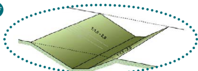
Vzorový příčný řez příkopem:
