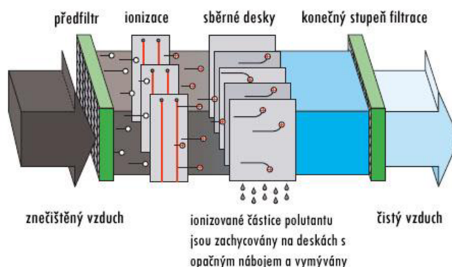
Obr. 8. – Elektrostatický filtr [13]
