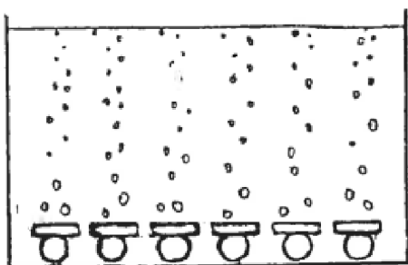
Obr. 17. – celoplošná aerace [19]
