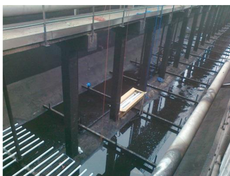
Foto č.2 – Demontáž stávajících aeračních elementů
