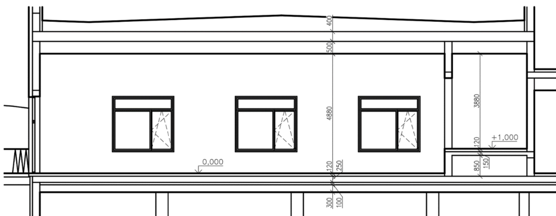
Obr. 3 Rez multifunkčnou sálou
