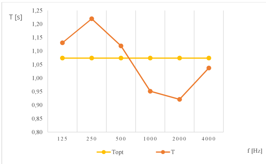
Graf 3 Priebeh vypočítanej doby dozvuku a optimálnej doby dozvuku na frekvencii - upravený stav
