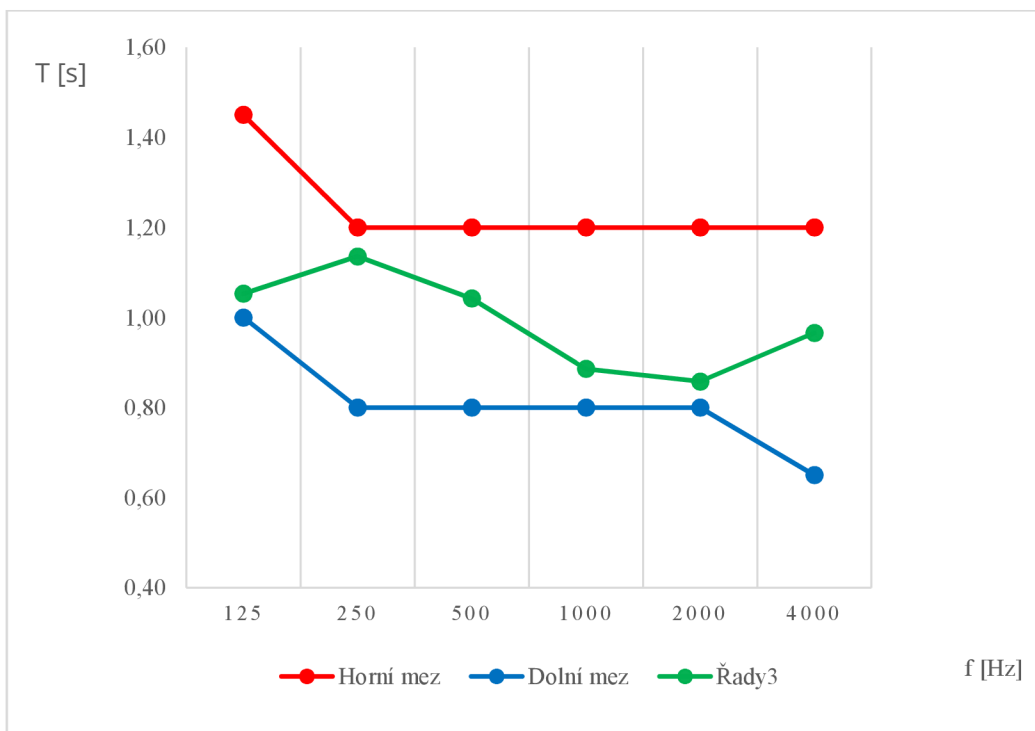
Graf 4 Priebeh vypočítanej doby dozvuku k optimálnej doby dozvuku na frekvencii - upravený stav
