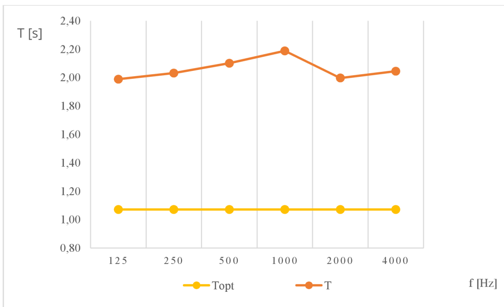
Graf 1 Priebeg vypočítanej doby dozvuku a optimálnej doby dozvuku na frekvencii – neupravený stav
