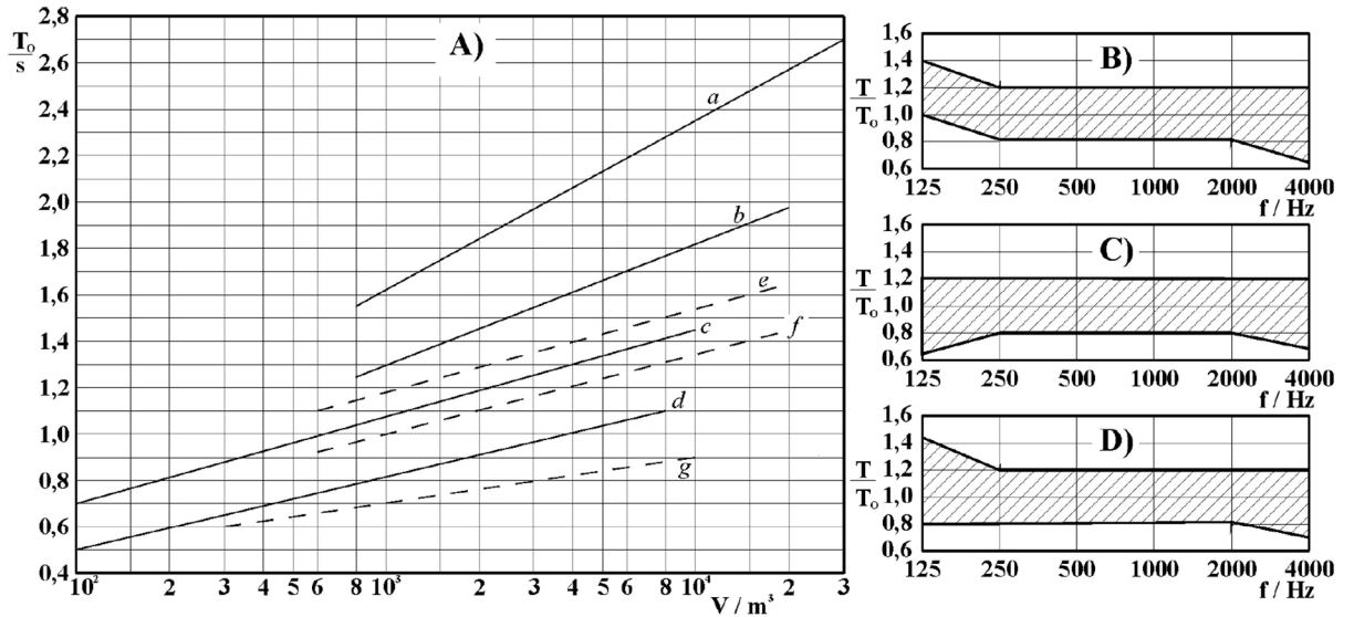
Obr. 1 A) Optimálna doba dozvuku T_{opt} [s] v závislosti na objeme a účele miestnosti [4]: a) Varhanná hudba, b) Orchestrálna hudba, c) Komorná hudba, d) Reč, e) Opera, f) Viacúčelové sály, g) Kíná; B) Dovolená tolerancia pre hudbu, C) Dovolená tolerancia pre reč a hudbu, D) Dovolená tolerancia pre reč
