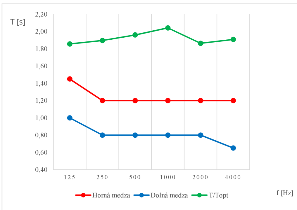
Graf 2 Priebeg vypočítanej doby dozvuku k optimálnej doby dozvuku na frekvencii – neupravený stav
