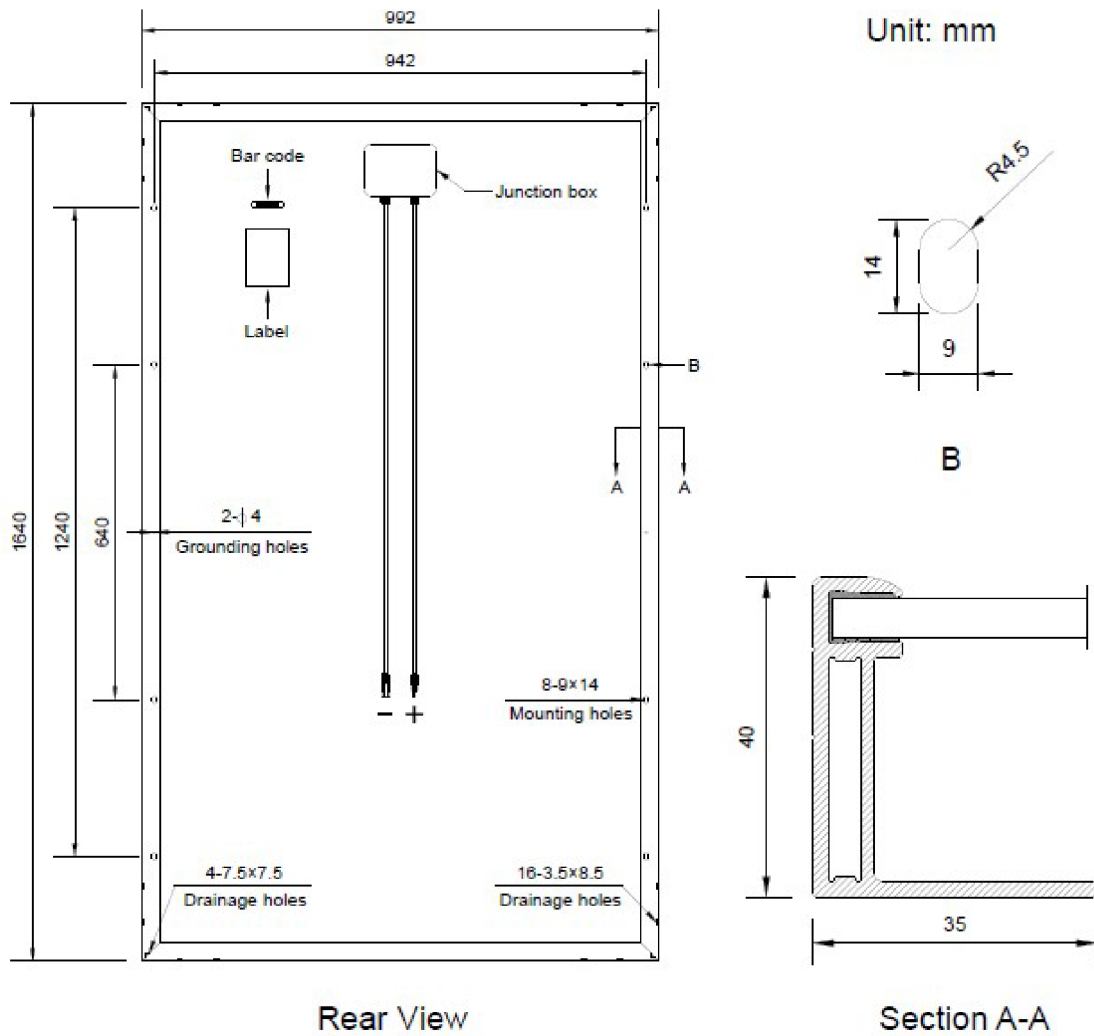
Obr. 1 Rozmery FV panelu [1]
