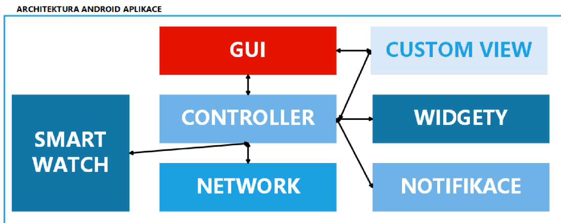
Obrázek 2.14: Schéma aplikace pro inteligentní domácnost v rámci projektu IoT pro platformu Android.
