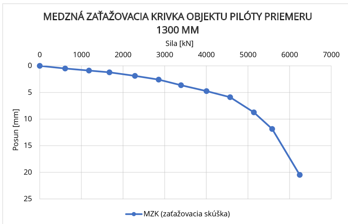
Graf 6.13 MZK objektu pilóty priemeru 1300 mm
