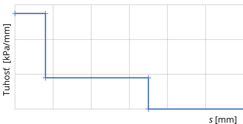
Graf 2.4 Zmena tuhosti vzhľadom k posunu pre FZ model
