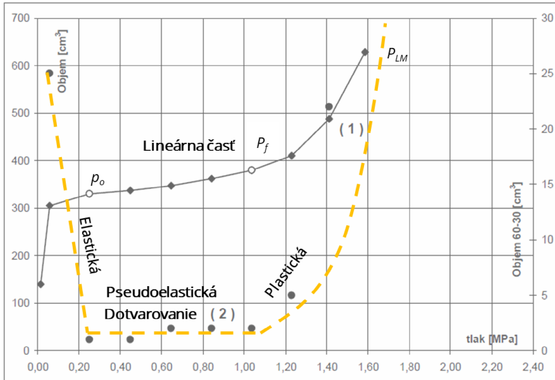
Obrázok 3.1 Schéma výstupu presiometrickej skúšky s jednotlivými fázami (Hudek, 2007) (SG-Geotechnika a.s., 2002)
