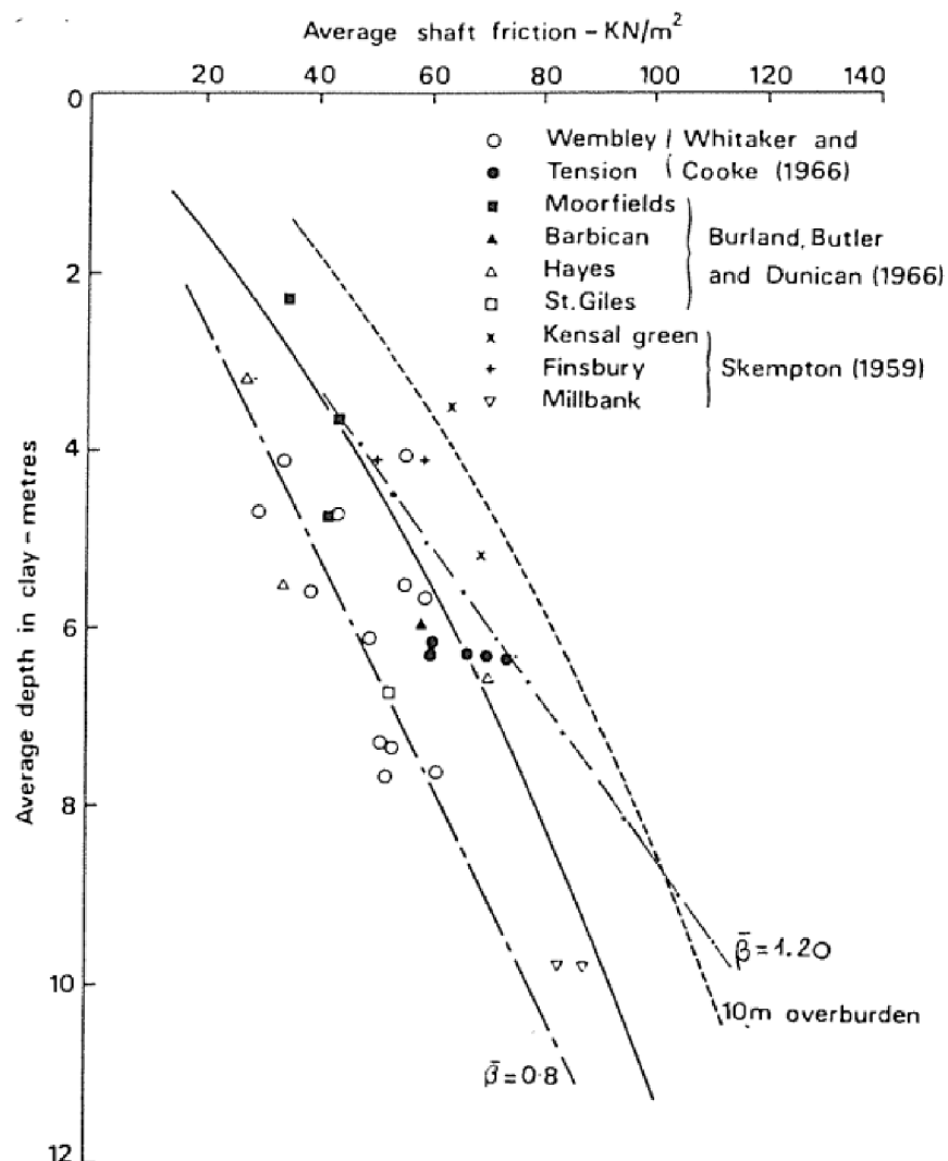
Obrázok 2.4 Závislosť medzného plášťového trenia na hĺbke (Burland, 1973) (Chalmrovský a kol., 2021)
