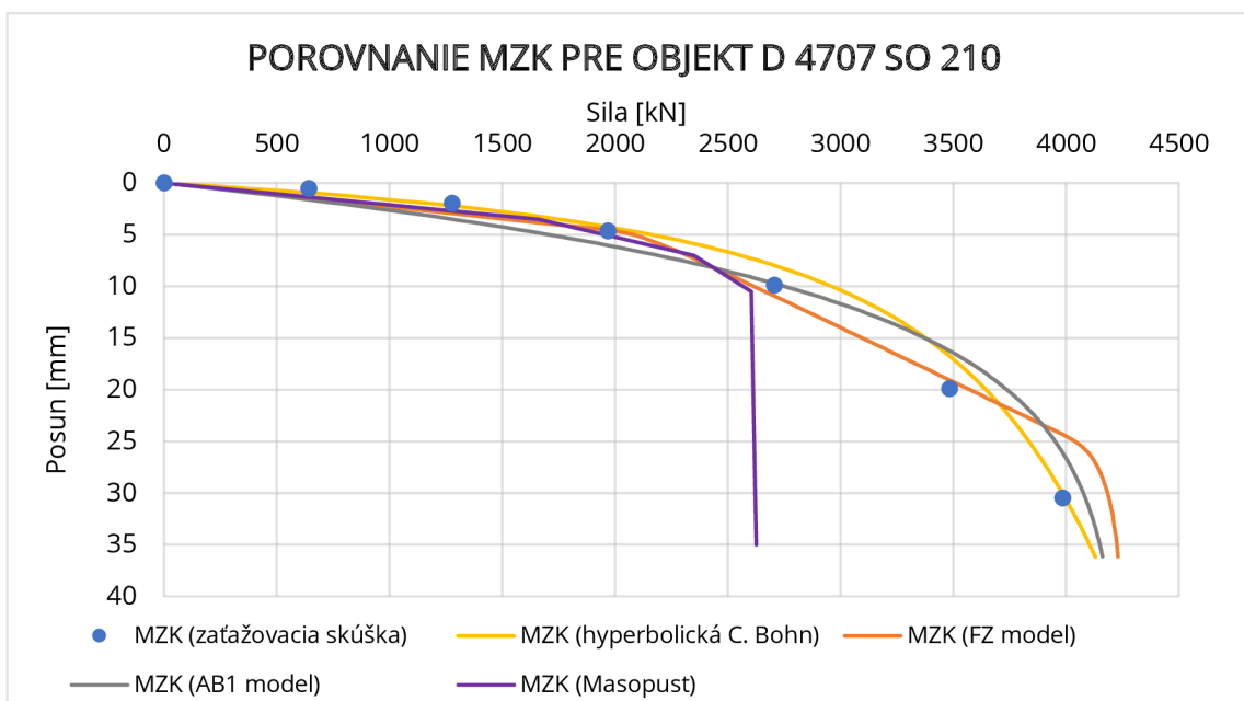
Graf 6.3 Porovnanie MZK pre objekt pilóty D 4707 SO 210
