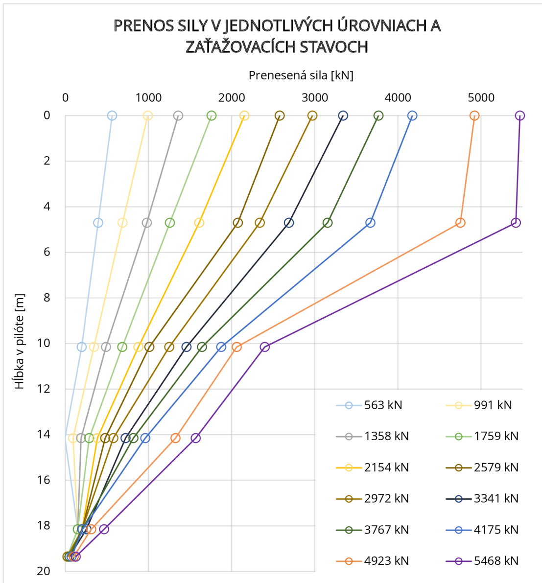
Graf 6.5 Prenos sily v jednotlivých zatažovacích stavoch po dĺžke objektu pilóty D 4704 SO 225
