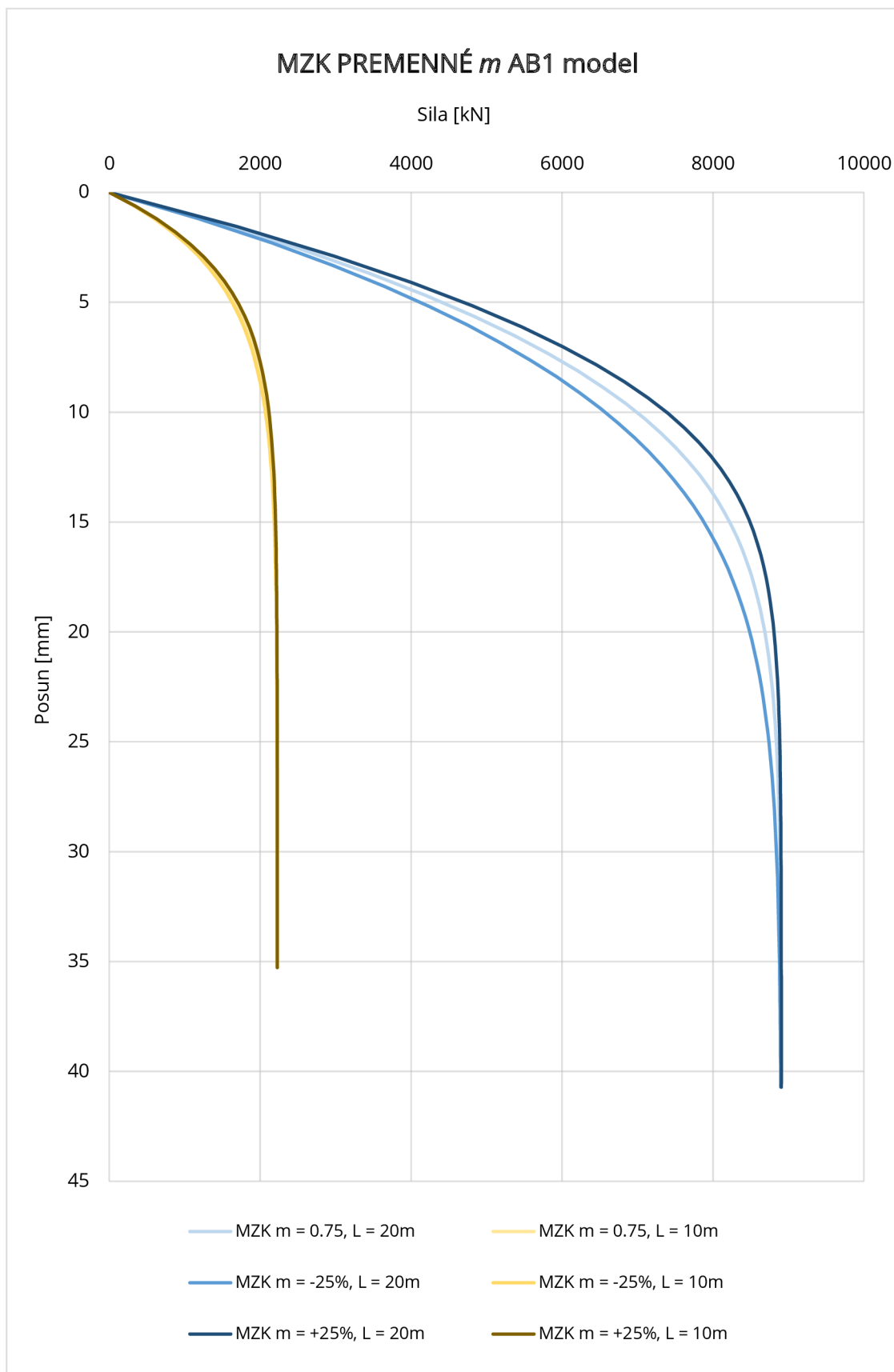
Graf 5.4 MZK AB1 modelu a premenného m
