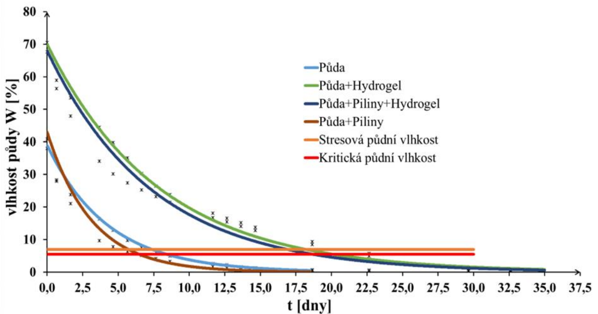
Obrázek 21: Změna půdní vlhkosti v jednotlivých variantách v čase experimentu.
