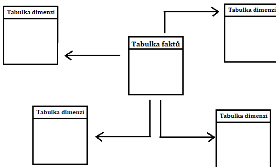
Obrázek 1.7:Hvězdicové schéma
