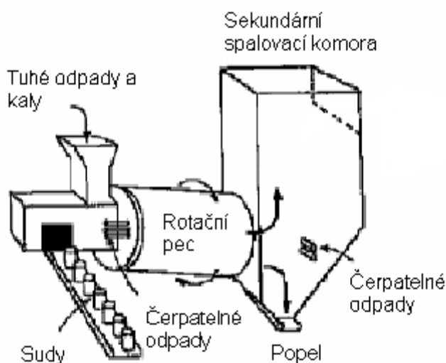
Obr. 10 Schéma spalovacího systému rotační pece [11]
