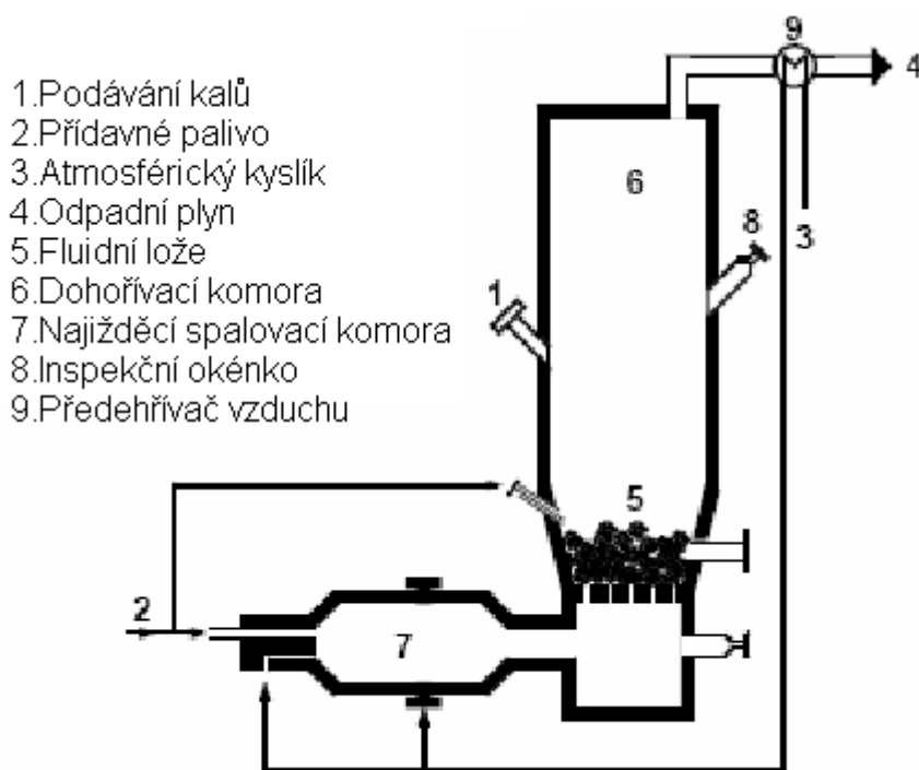
Obr. 11 Pevné resp. Probublávané fluidní lože [11]
