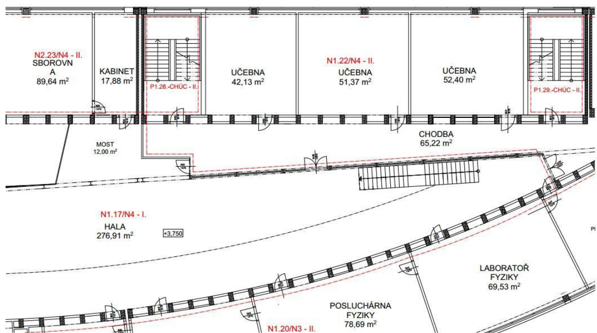
Obr. č. 7 - Změna dispozice přidáním chráněných únikových cest v typických NP
