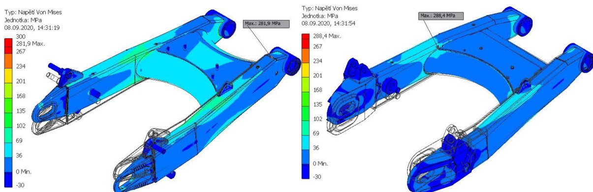
Obr. 26 Porovnání napětí při torzním zatížení ocelové vidlice (vlevo) a hliníkové vidlice (vpravo)
