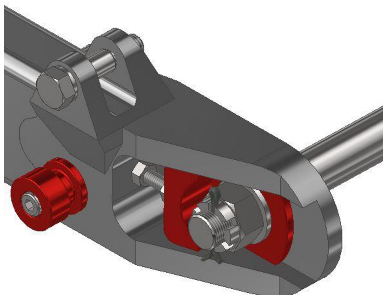
Obr. 16 Polohování osy kola, rolna a osa kola
