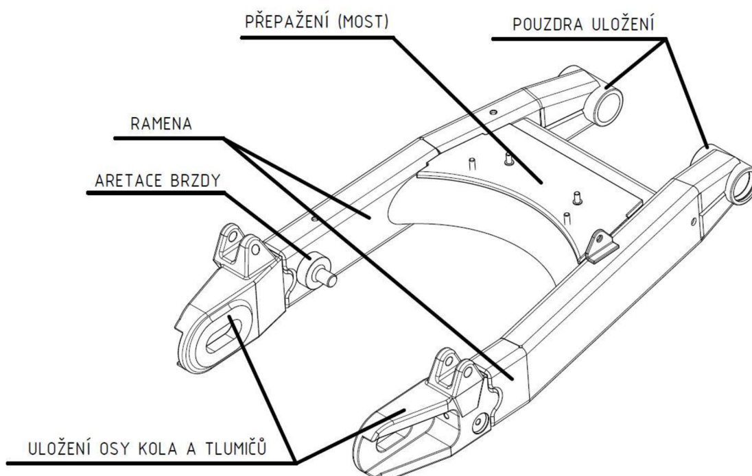
Obr. 3 Schéma kyvné vidlice
