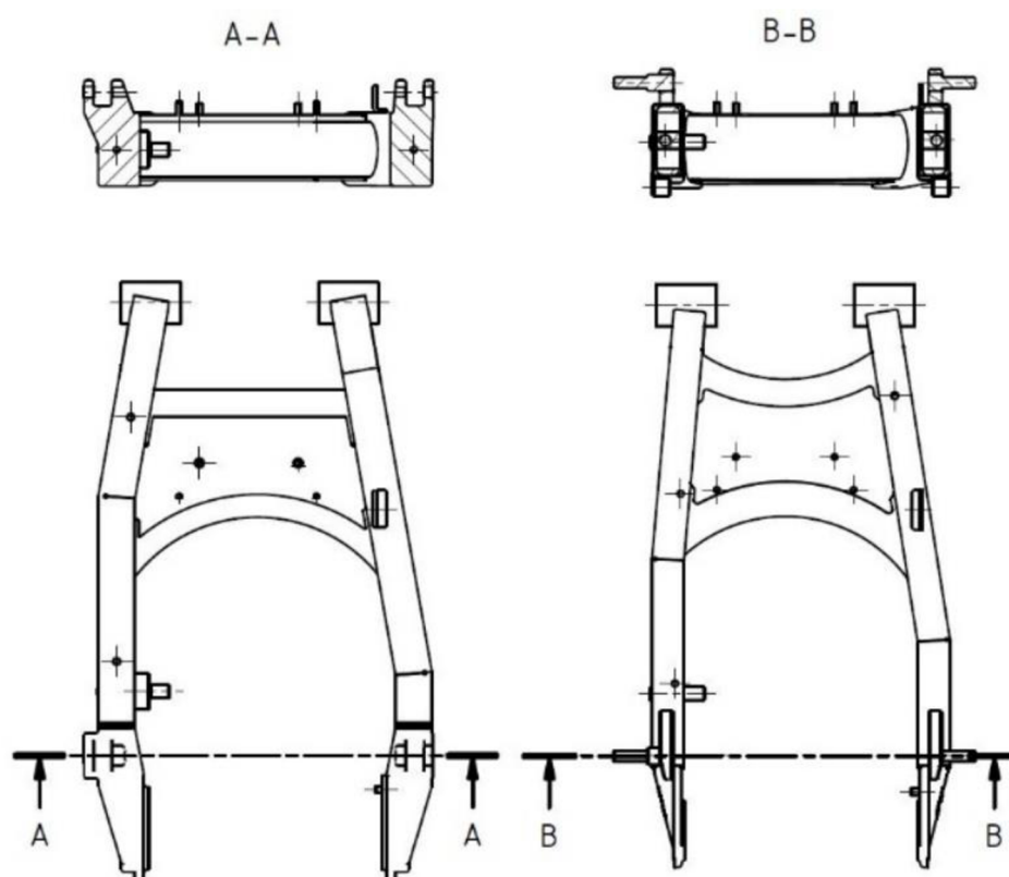
Obr. 27 Porovnání nové (vlevo) a původní vidlice (vpravo)
