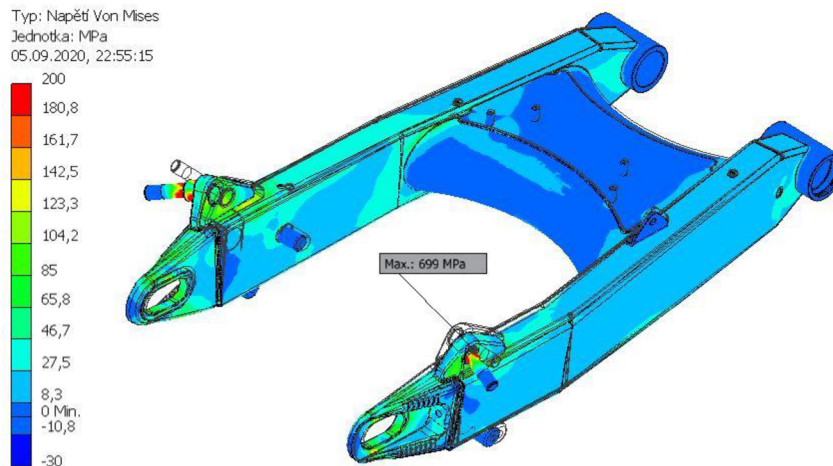
Obr. 22 Rozložení napětí u ocelové vidlice
