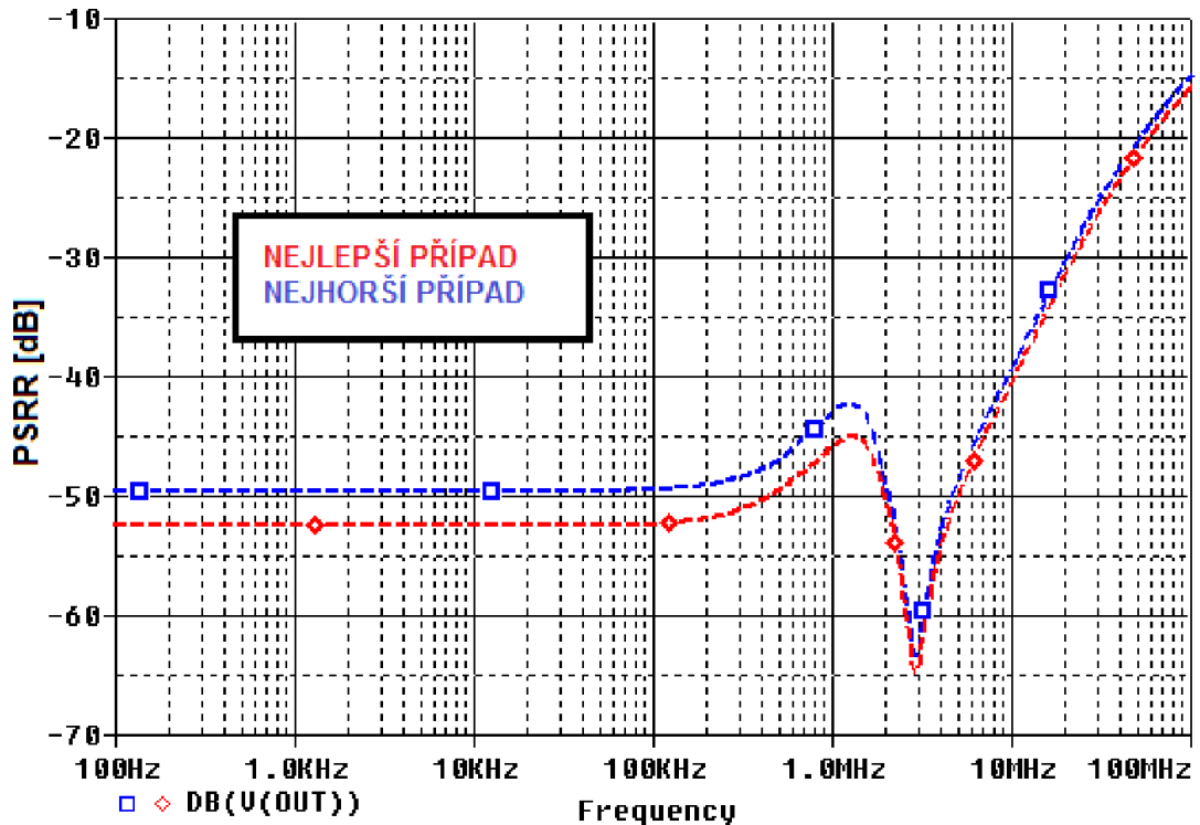
Obr. 4.30: PSRR LDO2, I_{ZATEZ} = 100 mA, nejhorší a nejlepší případ.
