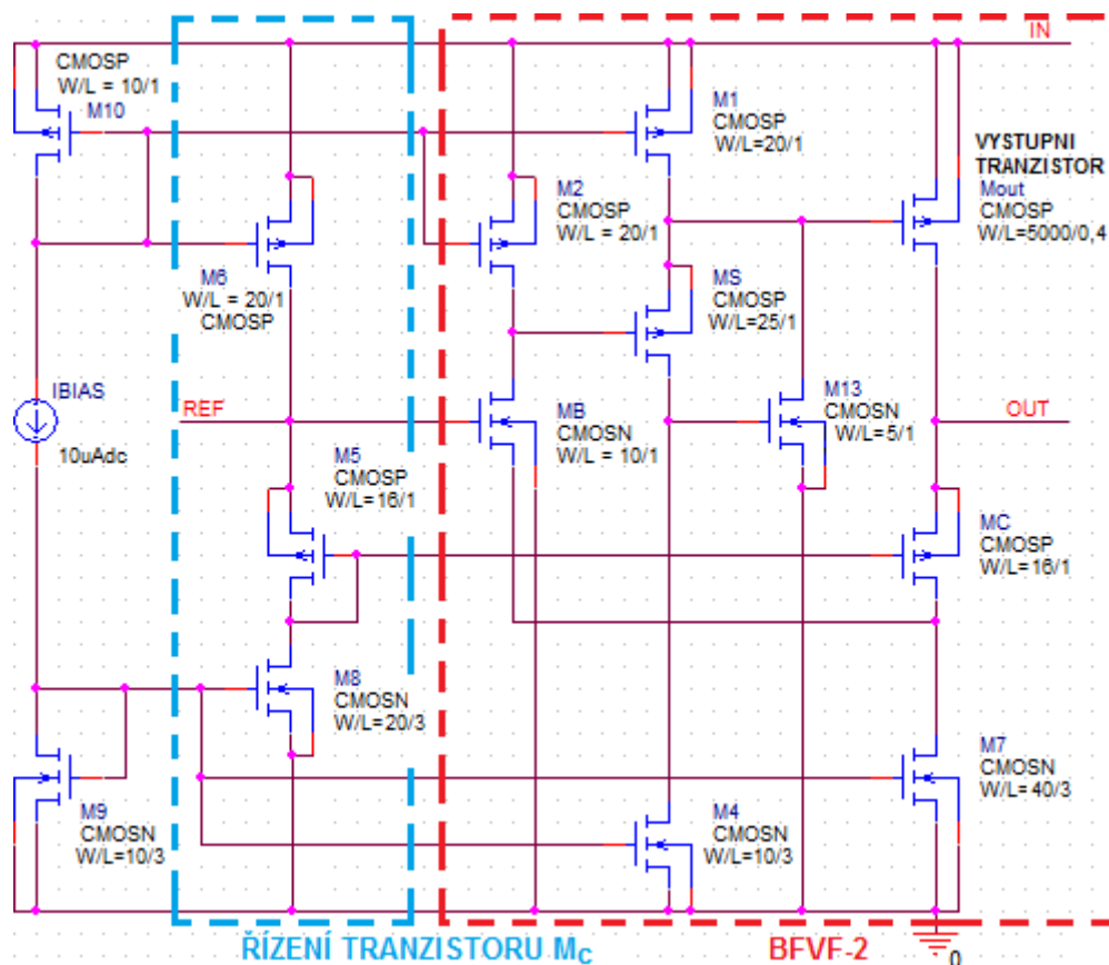
Obr. 4.76: Celkové schéma LDO4 se strukturou BFVF-2.
