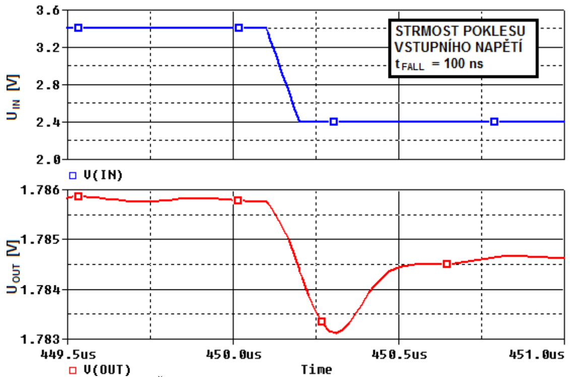
Obr. 4.22: Časová přechodná odezva LDO1 pro U_{IN} = 3,4 V \rightarrow 2,4 V.
