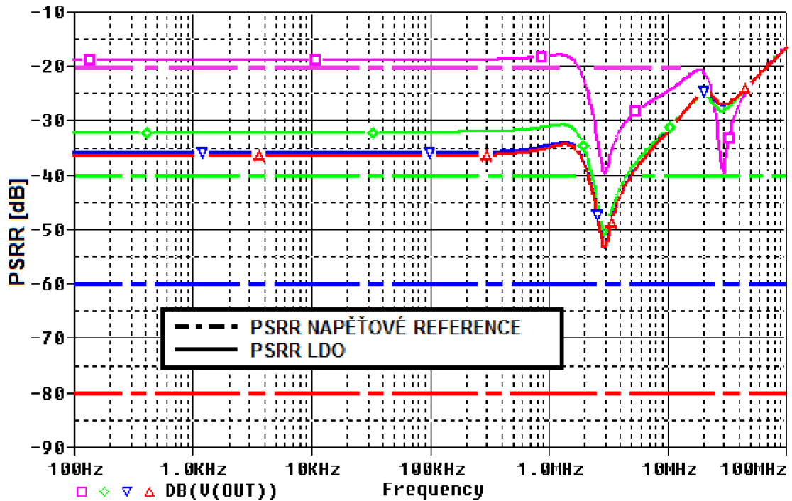
Obr. 4.75: PSRR LDO4 se strukturou BFVF-2, C_{OUT} = 1\mu\text{F} , U_{IN} = 2,4 \text{ V} , I_{ZATEZ} = 100 \text{ mA} , vliv neideální napěťové reference na PSRR LDO. \text{PSRR}_{REF} = -20 \text{ dB}; -40 \text{ dB}; -60 \text{ dB}; -80 \text{ dB} .
