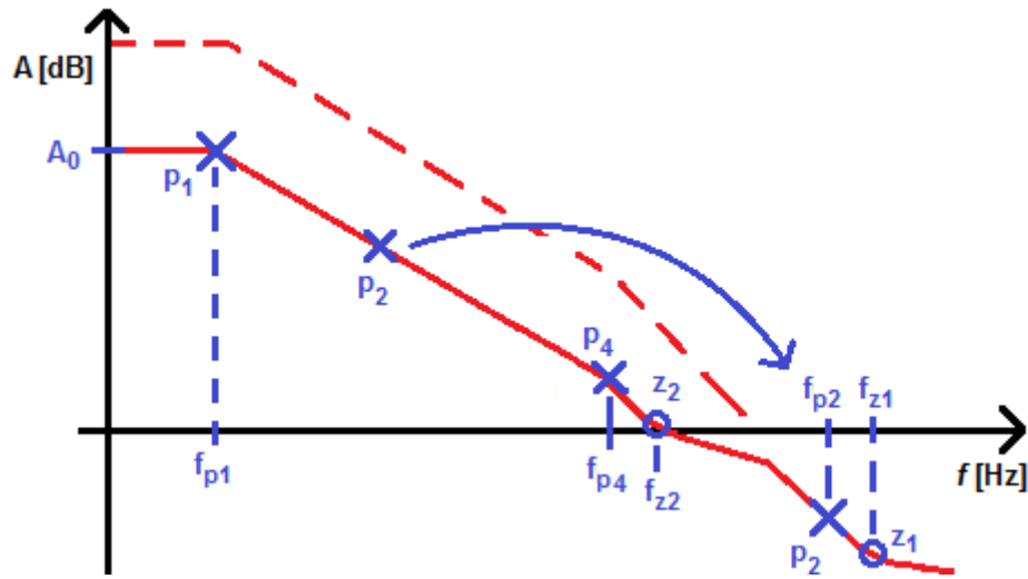
Obr. 4.7: Rozložení pólů a nul ve frekvenční charakteristice zisku zpětnovazební smyčky LDO1.
