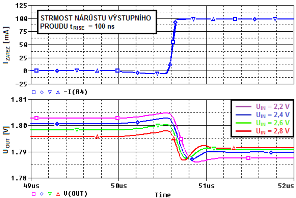
Obr. 4.79: Časová přechodná odezva LDO4 pro I_{ZATEZ} = 0 mA \rightarrow 100 mA.
