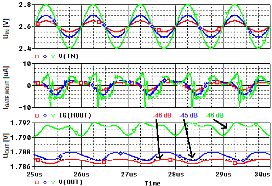
Obr. 4.104: Simulace potlačení vstupního zvlnění v časové oblasti, frekvence vstupního zvlnění 1 MHz, zvlnění \Delta U_{IN,PK-PK} = 100 mV; 200 mV, 400 mV.
