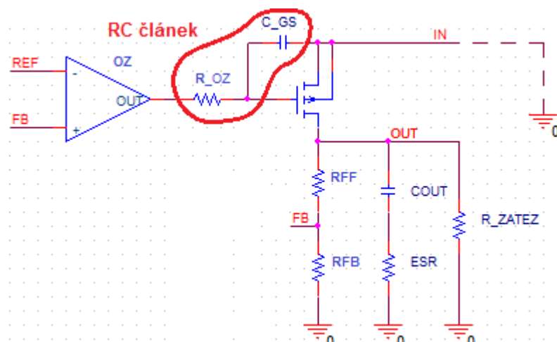
Obr. 4.3: Parazitní RC článek v zapojení LDO.
