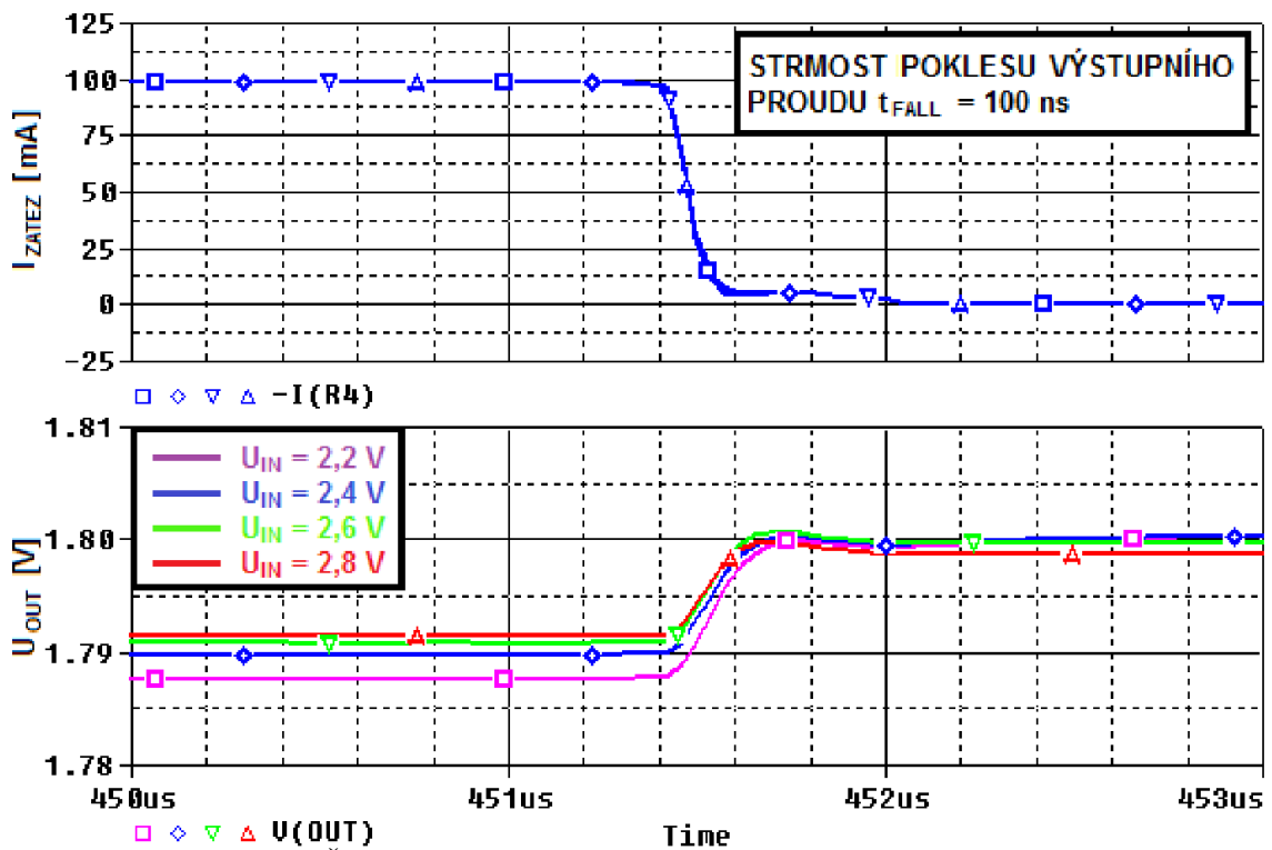
Obr. 4.80: Časová přechodná odezva LDO4 pro I_{ZATEZ} = 100 mA \rightarrow 0 mA.
