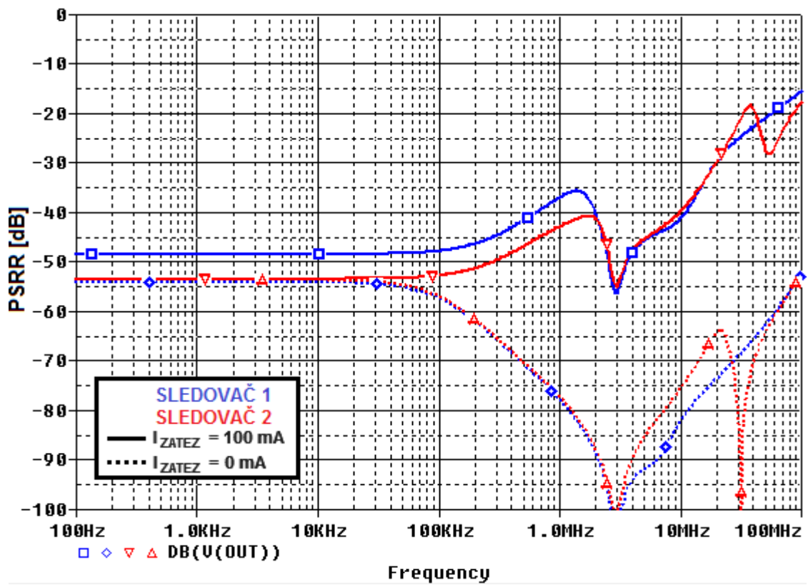
Obr. 4.49: PSRR LDO3 se sledovačem 1 a 2 pro I_{ZATEZ} = 100 \text{ mA} ; 0 \text{ A} .
