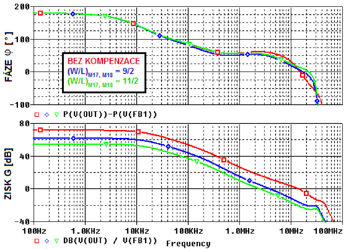
Obr. 4.47: Vliv kompenzace zisku diferenciálního stupně na charakteristiky zisku a fáze.
