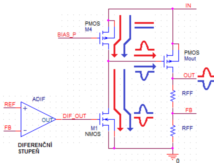
Obr. 4.83: Princip potlačení změn vstupního napětí klasického LDO.
