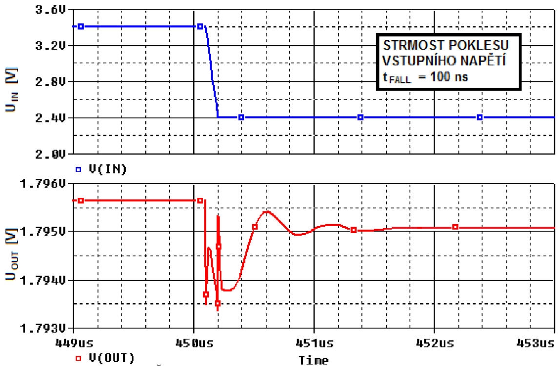
Obr. 4.35: Časová přechodná odezva LDO2 pro U_{IN} = 3,4 \text{ V} \rightarrow 2,4 \text{ V} .
