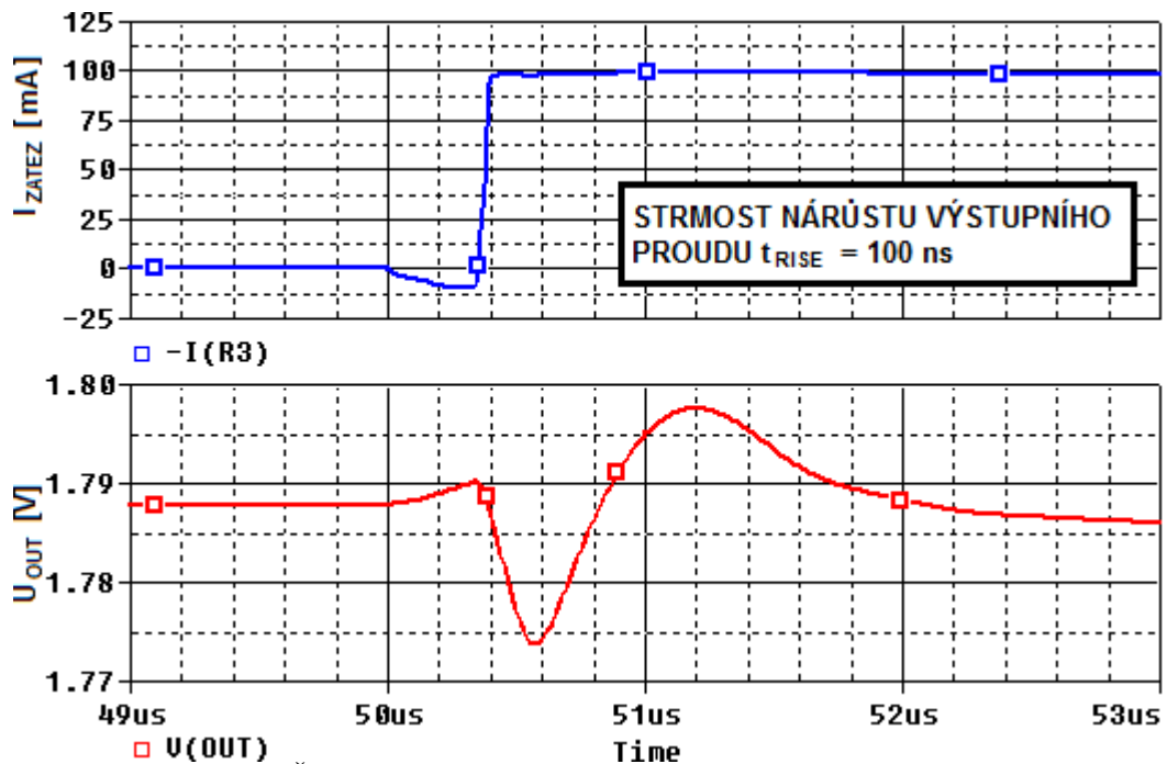
Obr. 4.105: Časová přechodná odezva LDO4 pro I_{ZATEZ} = 0 mA \rightarrow 100 mA.
