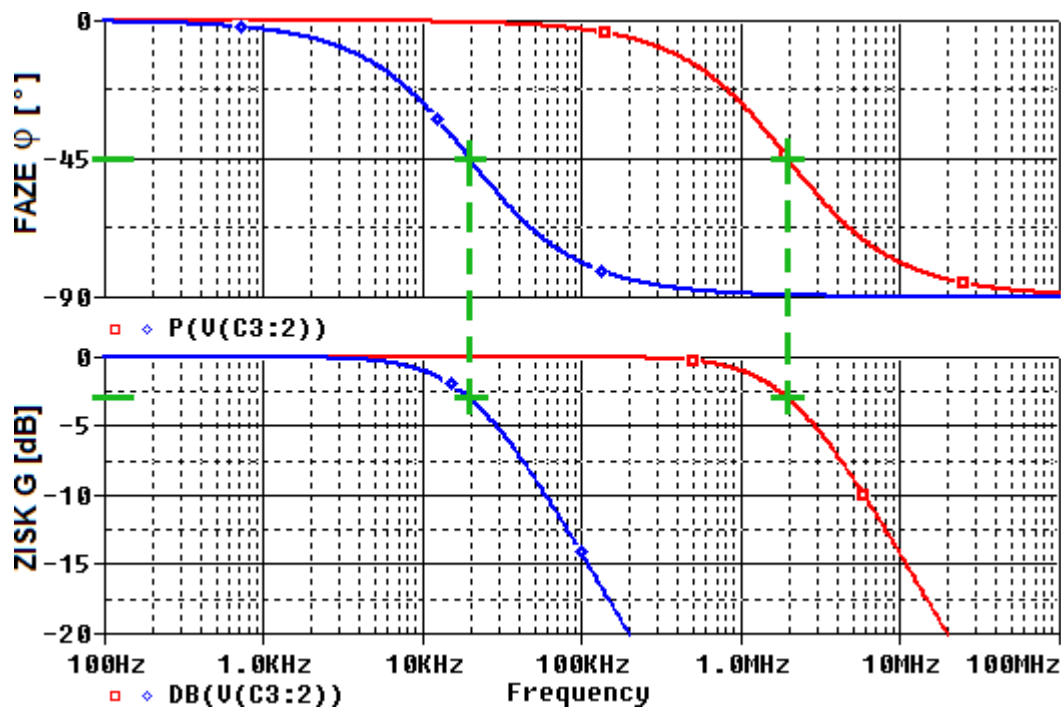
Obr. 4.4: Střídavá analýza zisku a fáze RC článku.
