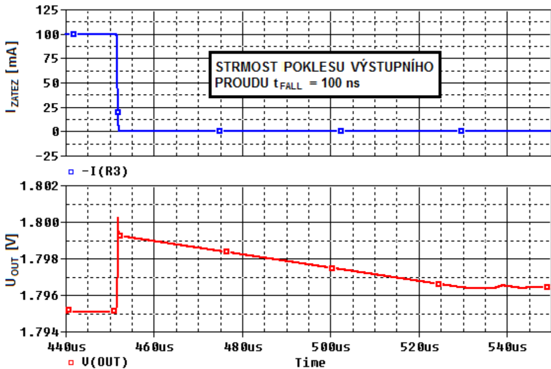
Obr. 4.37: Časová přechodná odezva LDO2 pro I_{ZATEZ} = 100 \text{ mA} \rightarrow 0 \text{ mA} .
