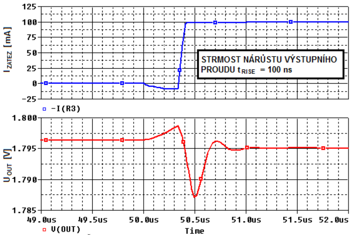
Obr. 4.36: Časová přechodná odezva LDO2 pro I_{ZATEZ} = 0 \text{ mA} \rightarrow 100 \text{ mA} .
