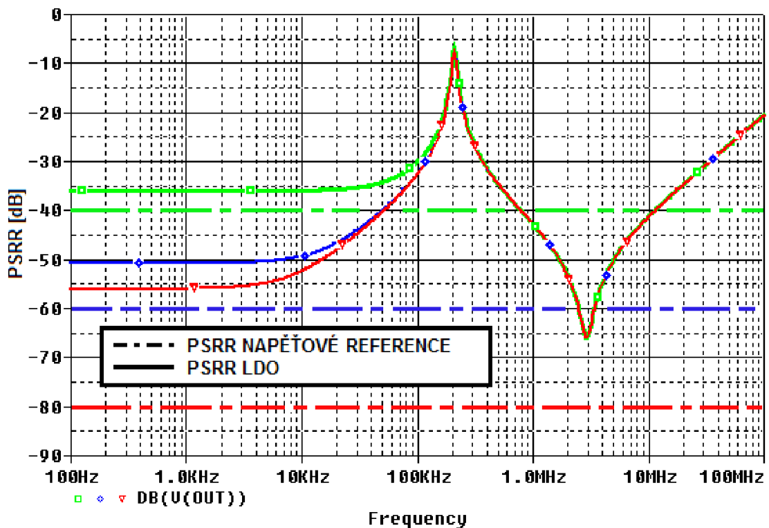
Obr. 3.8: Vliv neidální referencie na PSRR.
