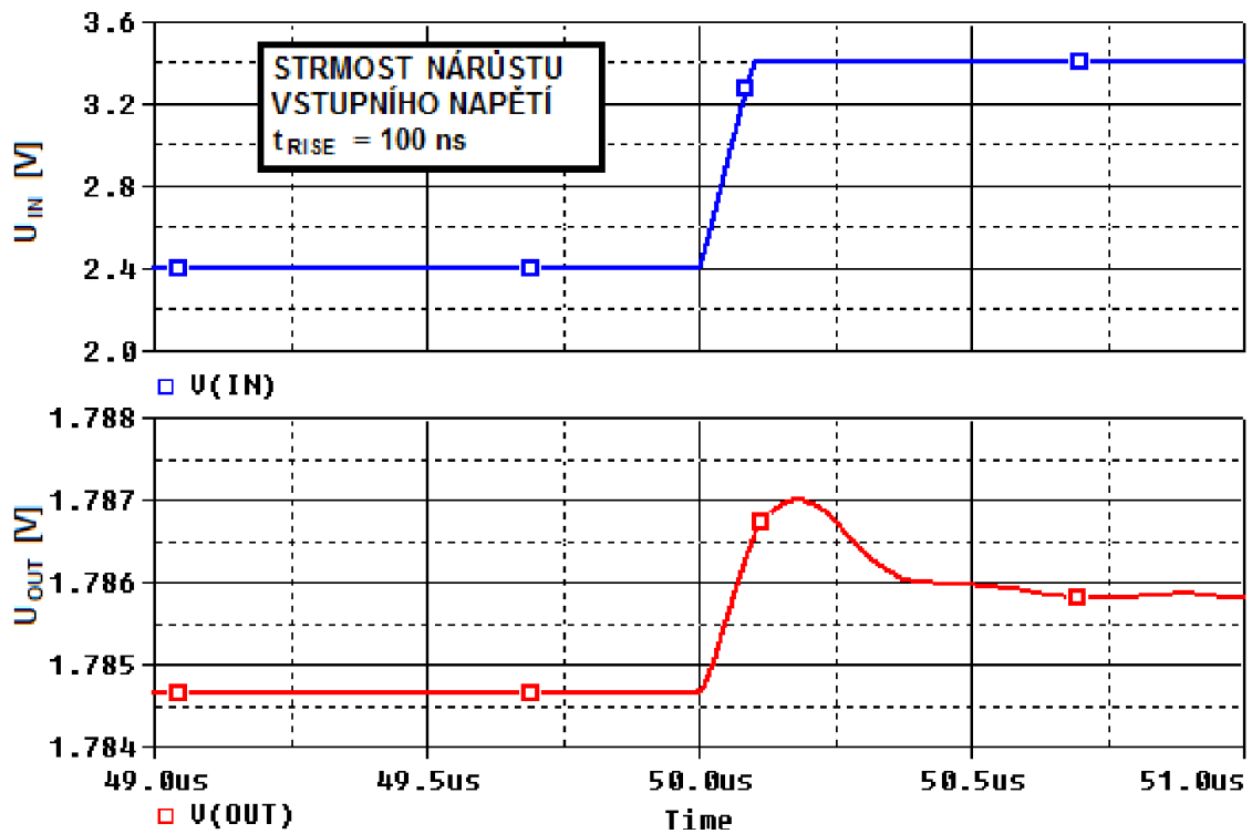
Obr. 4.21: Časová přechodná odezva LDO1 pro U_{IN} = 2,4 V \rightarrow 3,4 V.
