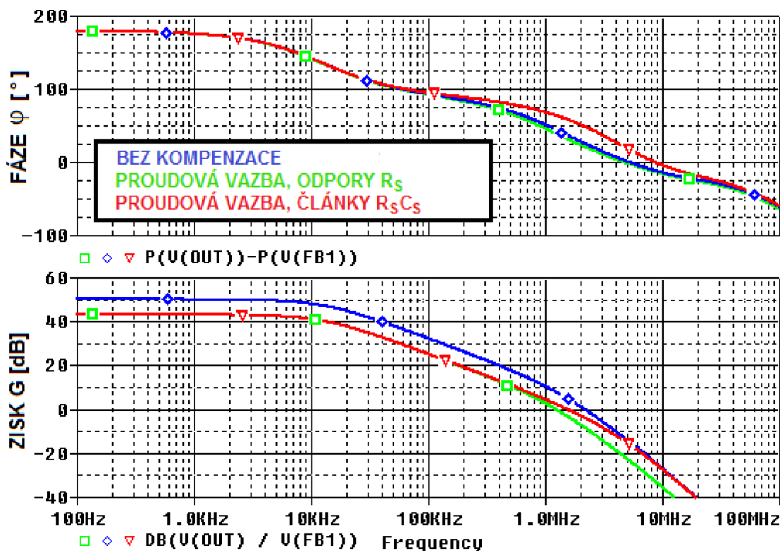
Obr. 4.12: Vliv R_S C_S článku na zisk a fáze otevřené smyčky LDO s proudovou vazbou 1 pro I_{ZATEZ} = 100 mA.
