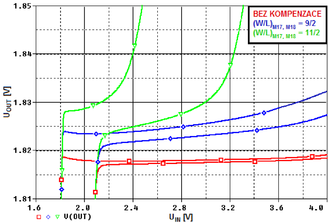
Obr. 4.48: Vliv kompenzace zisku diferenciálního stupně na parametry \Delta U_{OUT}/\Delta I_{ZATEZ} a \Delta U_{OUT}/\Delta U_{IN} .
