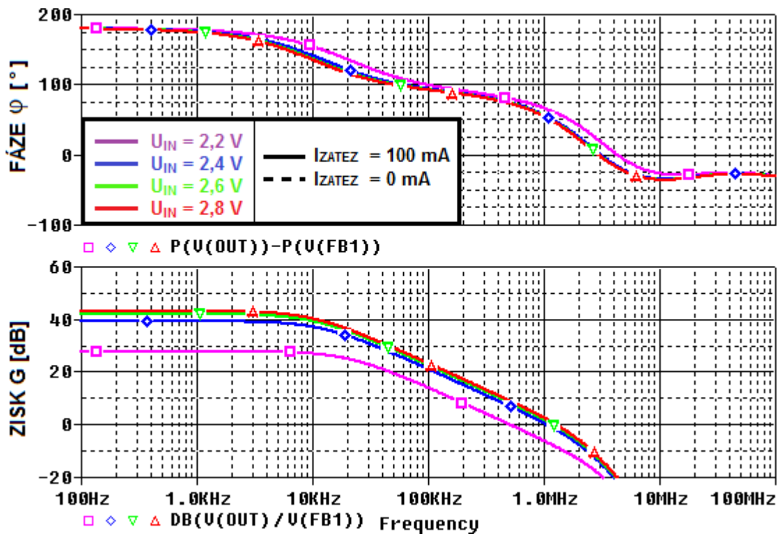
Obr. 4.68: Zisk a fáze LDO3 se strukturou BFVF, I_{ZATEZ} = 100\text{ mA} ; 0A U_{IN} = 2,2\text{ V} ; 2,4 V 2,6 V; 2,8 V.
