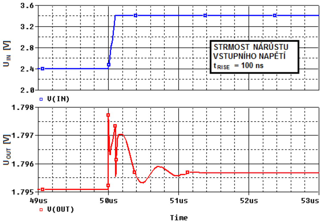
Obr. 4.34: Časová přechodná odezva LDO2 pro U_{IN} = 2,4 \text{ V} \rightarrow 3,4 \text{ V} .
