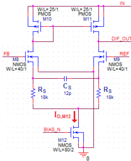
Obr. 4.84: Diferenční stupeň.
