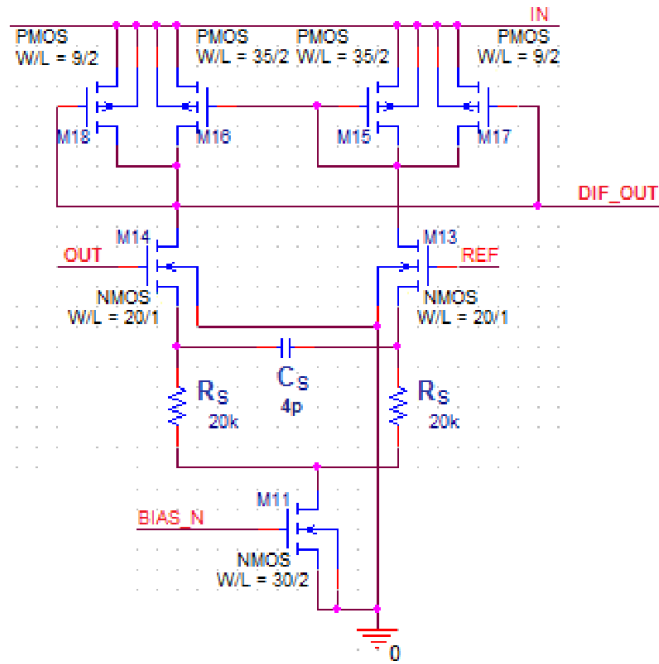
Obr. 4.46: Frekvenční kompenzace zisku diferenčního páru.
