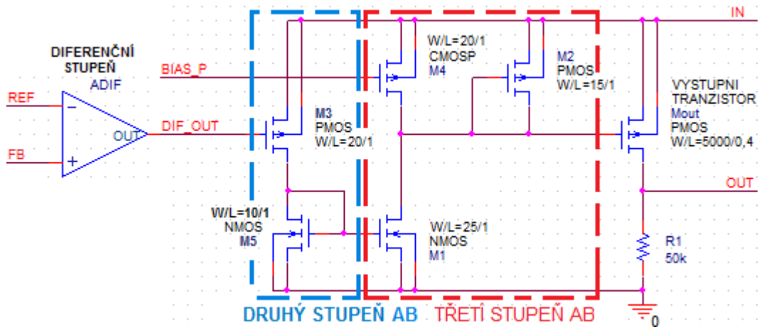
Obr. 4.25: Třetí stupeň ve třídě AB s posunem vstupní úrovně.
