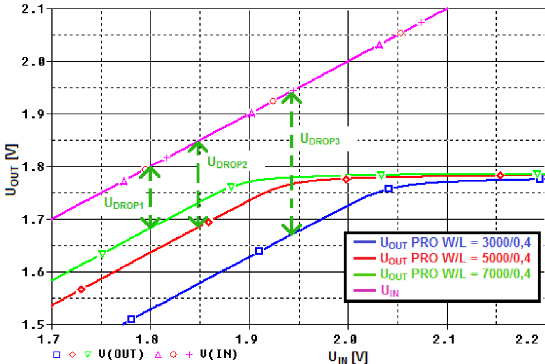
Obr. 4.2: Převodní charakteristika LDO a napětí U_{DROP} při I_{ZATEZ} = 100 mA.
