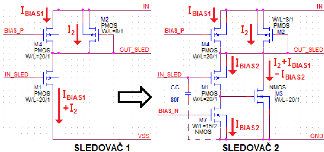
Obr. 4.41: Schema sledovače 3.
