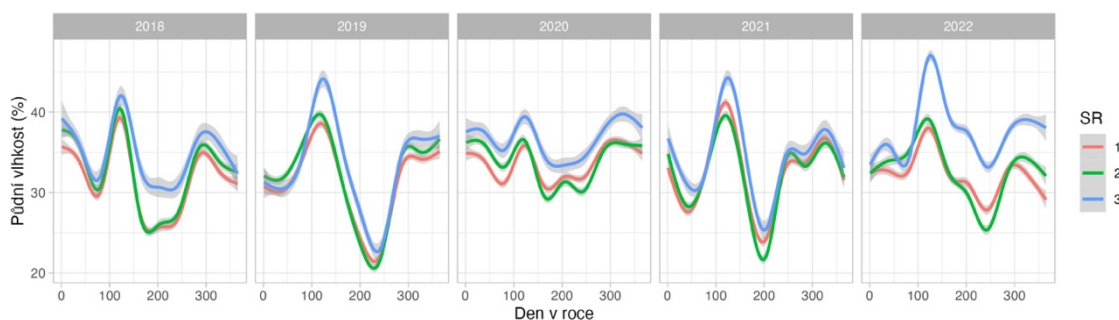
Obrázek 10. GAM model zobrazující vývoj půdní vlhkosti v porostech s různým počtem druhů dřevin v závislosti na čase v letech 2018 až 2022. Linie znázorňují nabitovaný GAM model a šedá zóna kolem nich 95% intervaly spolehlivosti.
