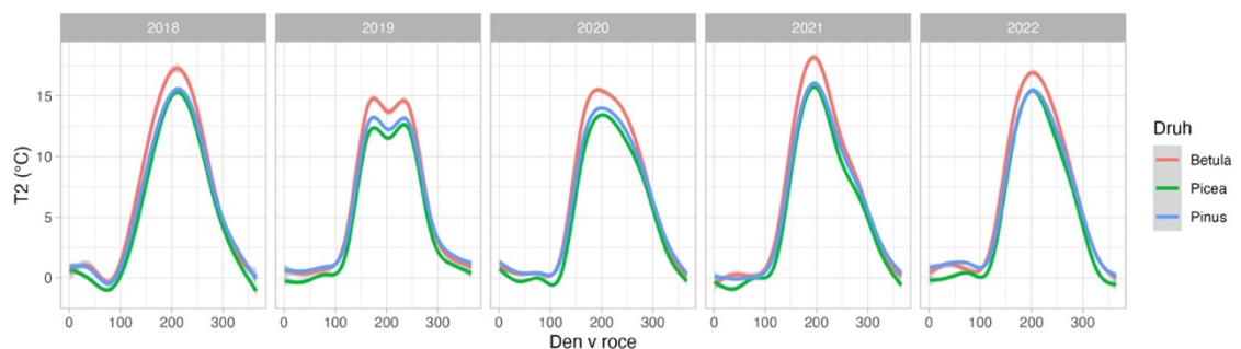
Obrázek 22. GAM model zobrazující vývoj teploty T2 v monokulturách borovice ( Pinus ), břízy ( Betula ) a smrku ( Picea ) v závislosti na čase v letech 2018 až 2022. Linie znázorňují nafitovaný GAM model a šedá zóna kolem nich 95% intervaly spolehlivosti.
