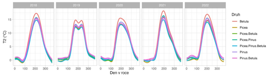
Obrázek 26. GAM model zobrazující vývoj teploty T_2 v porostech s různou druhovou skladbou dřevin v závislosti na čase v letech 2018 až 2022. Linie znázorňují nafitovaný GAM model a šedá zóna kolem nich 95% intervaly spolehlivosti.
