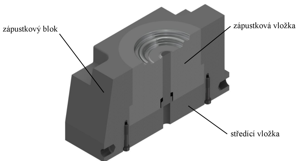
Obr. 56 Vložkování zápustky
