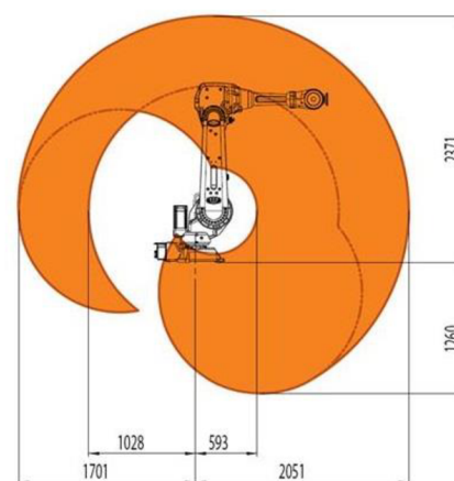
Obr. 68 Pracovní prostor [52]
