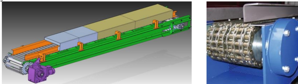
Obr. 32 Řetězový dopravník [36], [37]
