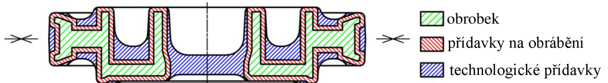
Obr. 47 Přídávky
