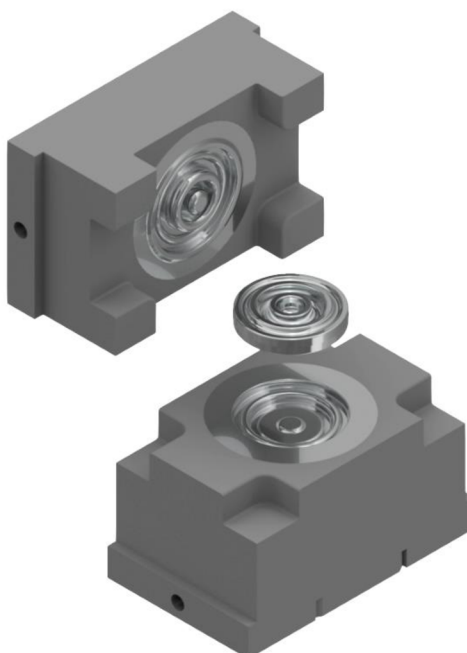
Obr. 59 Vizualizace sestavy předkovací zápusky
