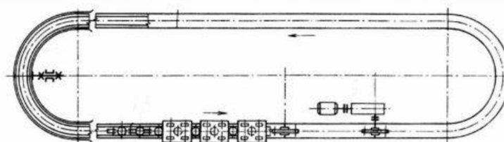
Obr. 35 Okružní dopravník [40]
