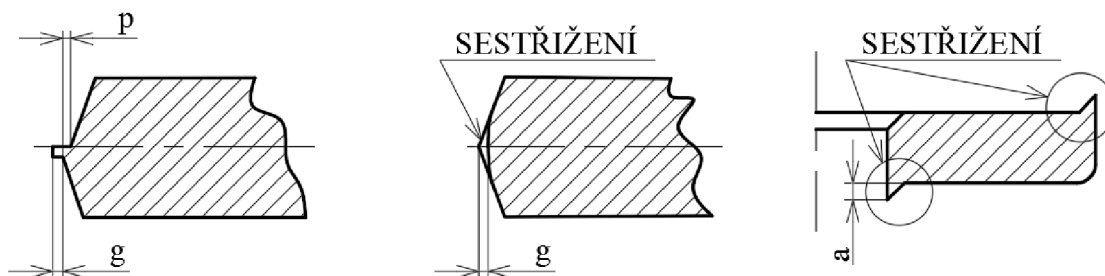
Obr. 48 Úchylky tvaru výkovku [18]
