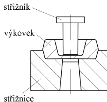
Obr. 19 Děrování [2]
