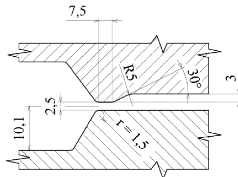
Obr. 50 Rozměry drážky
