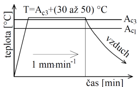
Obr. 20 Normalizační žihání [24]
