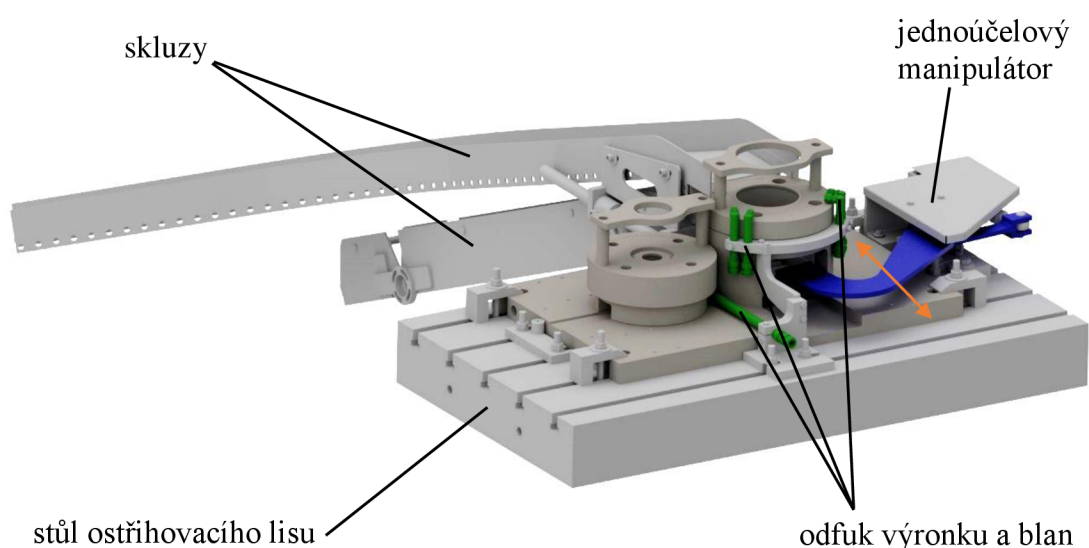
Obr. 72 Stůl ostříhovacího lisu (vizualizace Inventor 2019)
