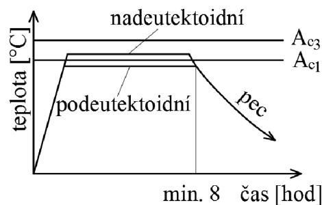
Obr. 21 Žihání na měkko [24]
