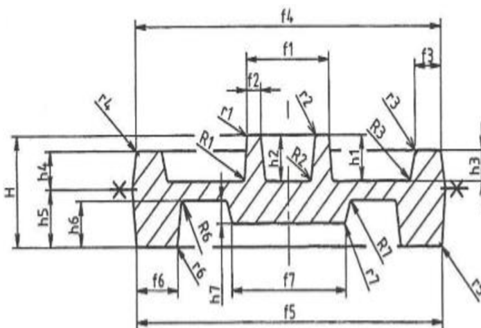
Obr. 11 Zaoblení hran výkovku [19]
