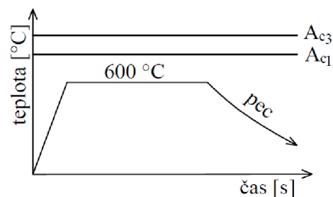
Obr. 22 Žihání ke snížení pnutí [24]
