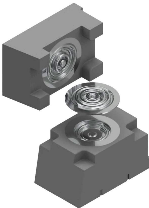
Obr. 58 Vizualizace sestavy dokončovací zápusky
