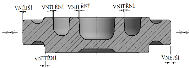
Obr. 44 Úkosy
