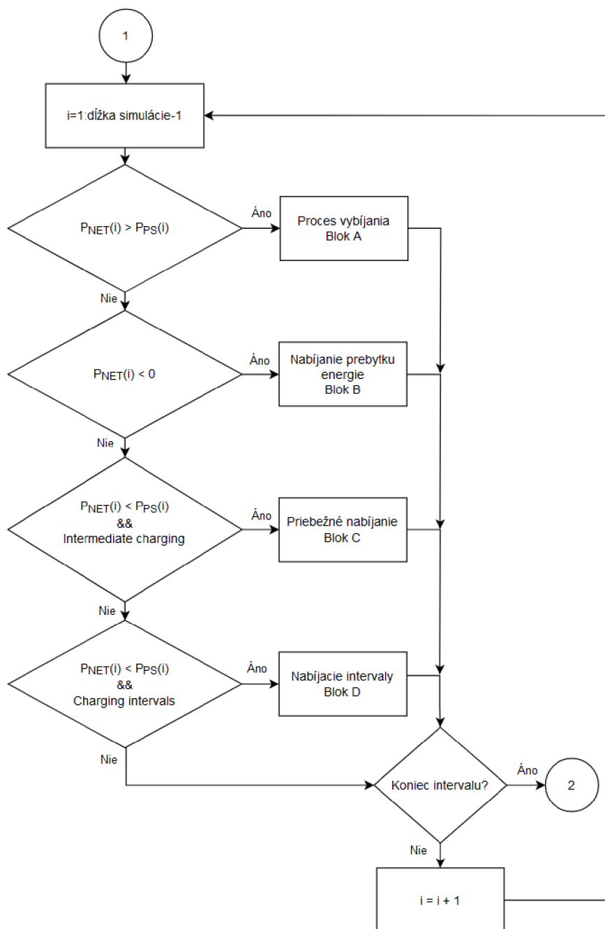
Obrázok 16: Vývojový diagram algoritmu pre riadenie vybíjania a nabíjania batériového úložiska
