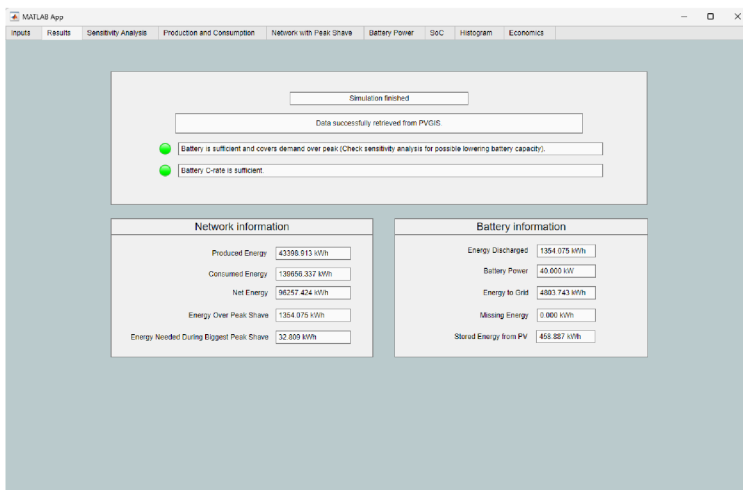
Obrázok 30: Rozloženie karty s výsledkami simulácie
