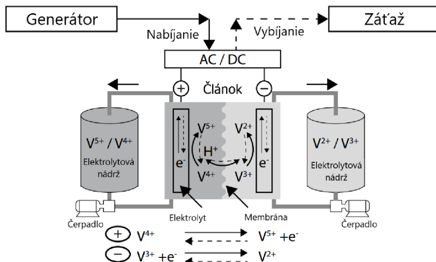
Obrázok 5: Schematický diagram prietokovej batérie [4]
