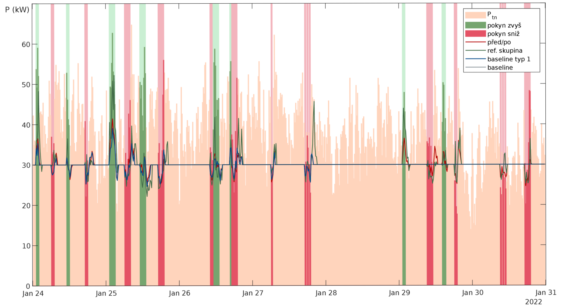
Obr. 6.1: průběh poměrné změny zatížení 24. 01. 2022–30. 01. 2022
