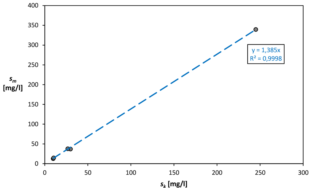
Obr. 49. Analýza závislosti s_m na s_k , vodoměrný profil Přebice
