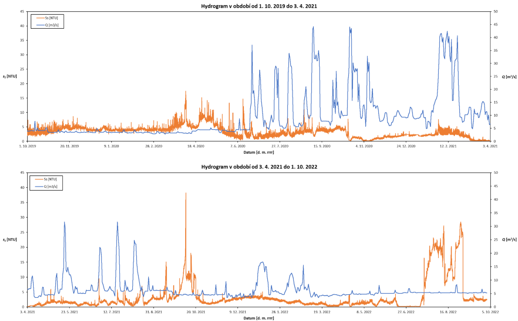
Obr. 63. Hydrogram vzniklý metodou korekce dat pomocí vyhlazení a doplnění, vodoměrný profil Znojmo
