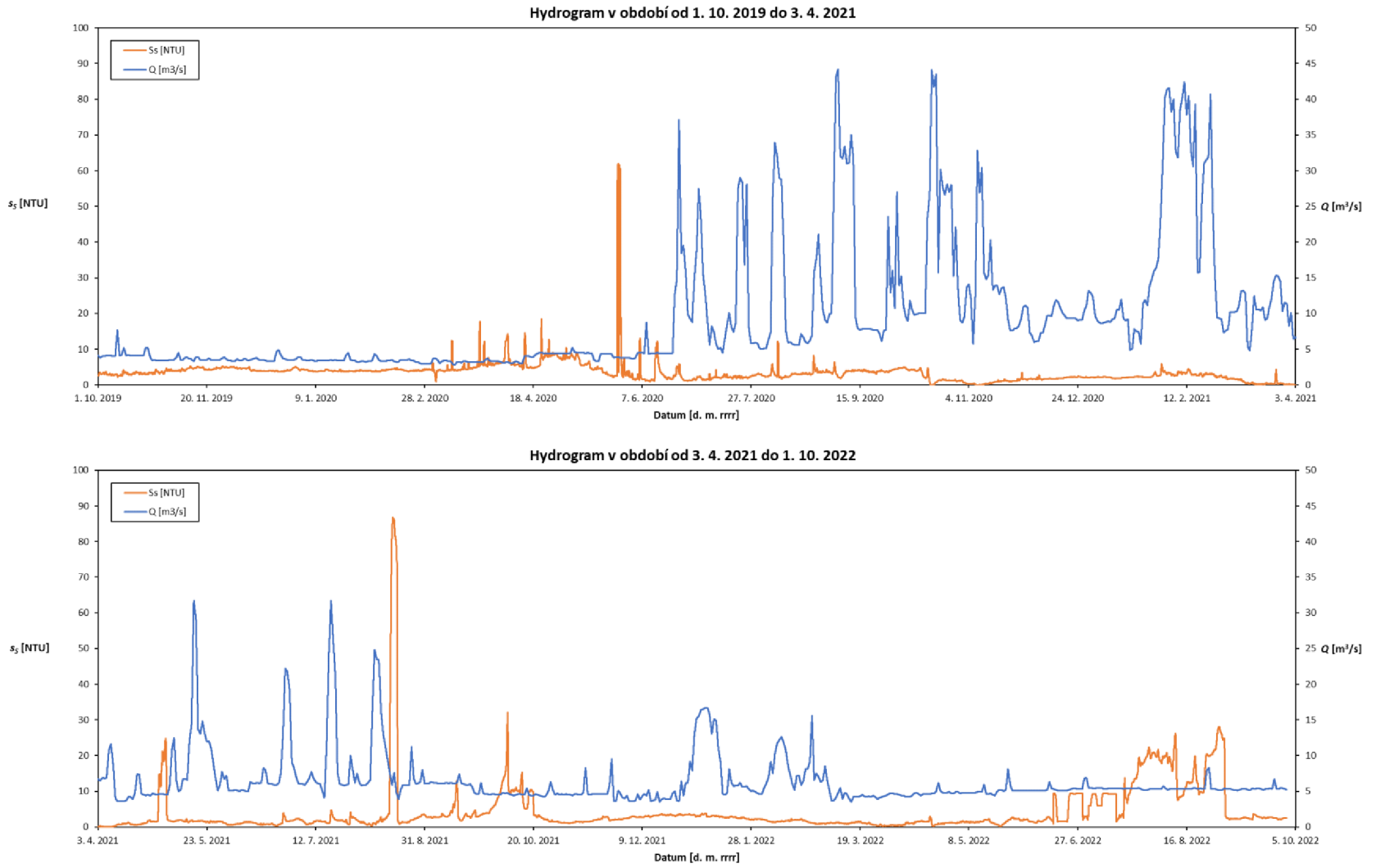
Obř. 65. Hydrogram vzniklý metodou korekce dat pomocí UNS, vodoměrný profil Znojmo
