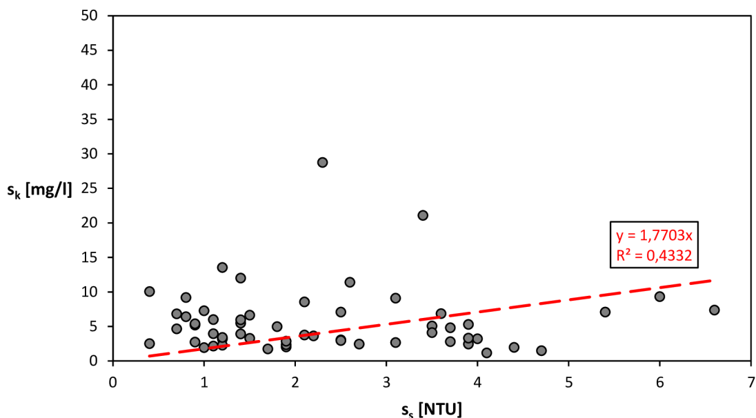
Obr. 68. Kalibrace sondy v obci Znojmo
