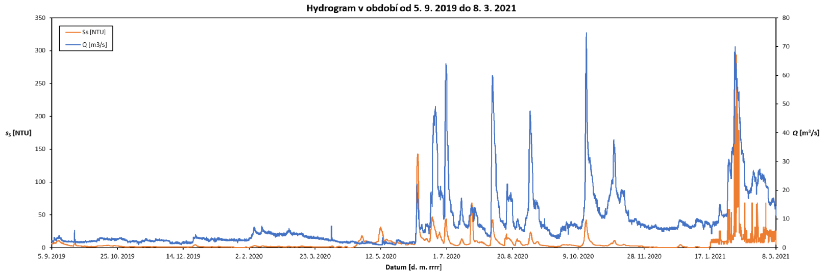
Obř. 47. Hydrogram vzniklý metodou korekce dat pomocí UNS, vodoměrný profil Přibice
