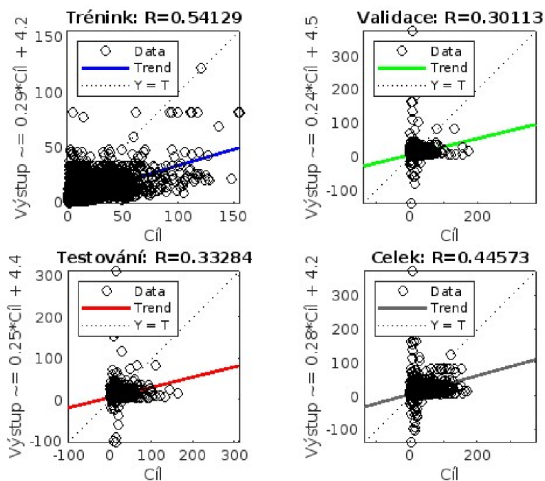
Obr. 36. Spolehlivost testovací UNS složené z 1 000 skrytých neuronů, vytvořeno pro vodoměrný profil Hevlín
