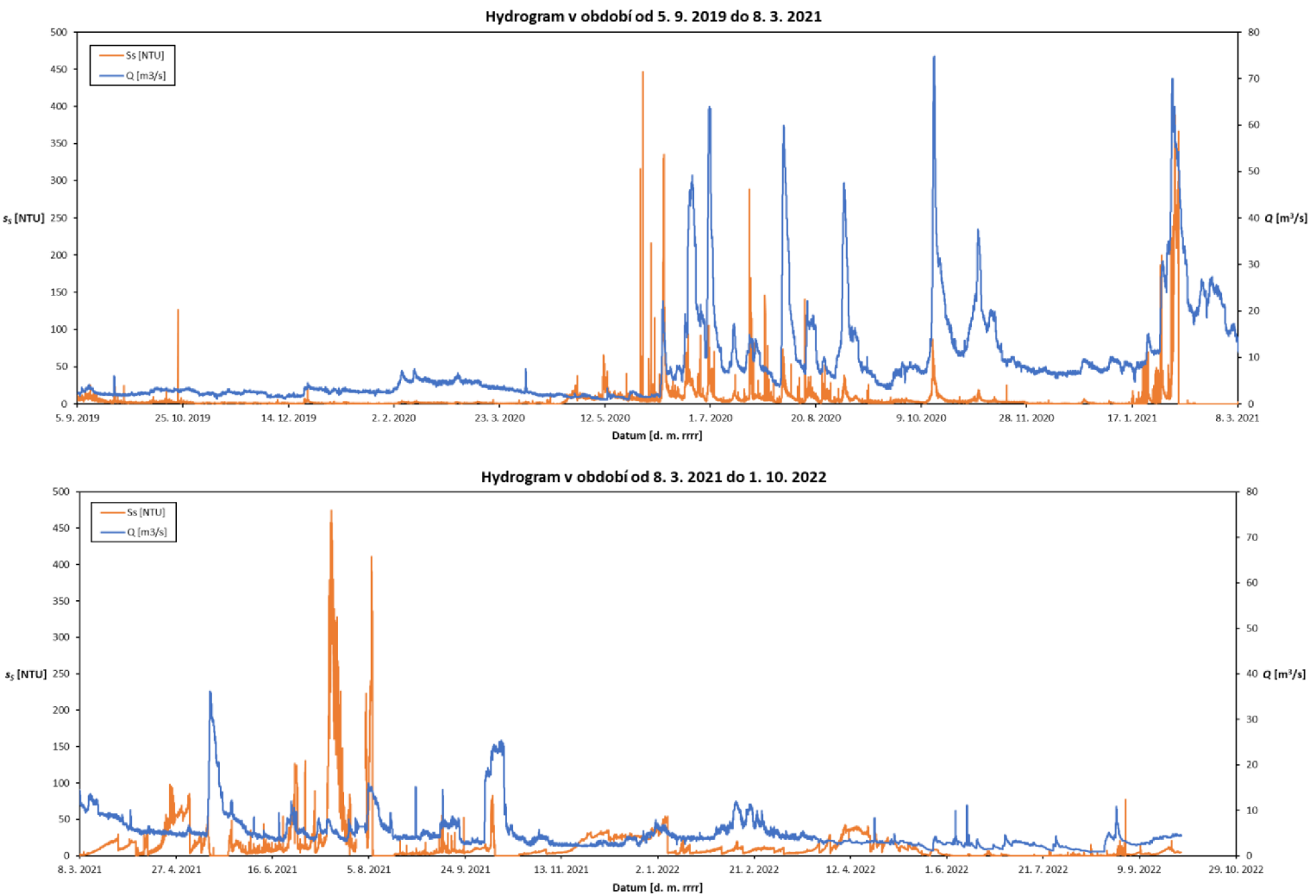
Obr. 42. Hydrogram vzniklý metodou bez korekce dat, vodoměrný profil Přibice
