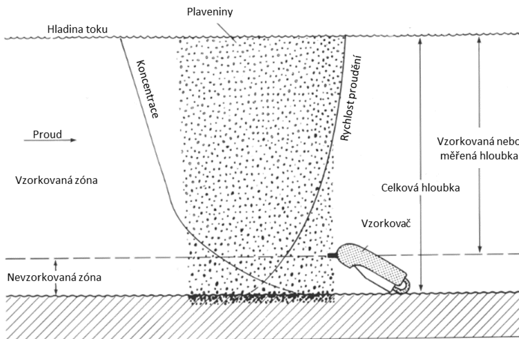
Obr. 9. Vzorkovaná a nevzorkovaná zóna v odběrové vertikále s ohledem na rychlost proudění a koncentraci suspendovaných látek [9]
