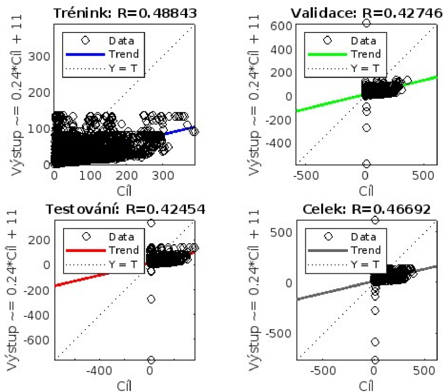
Obr. 55. Spolehlivost natrénované UNS vytvořené pro vodoměrný profil Židlochovice
