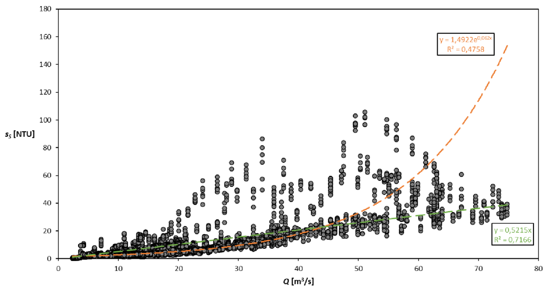
Obr. 44. Korelace mezi vybranými hodnotami s_s a odpovídajícími Q ve vodoměrném profilu Přibice
