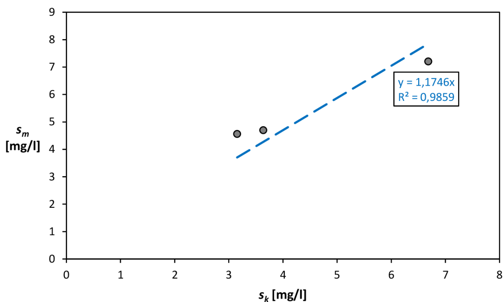
Obr. 67. Analýza závislost s_m na s_k , vodoměrný profil Znojmo
