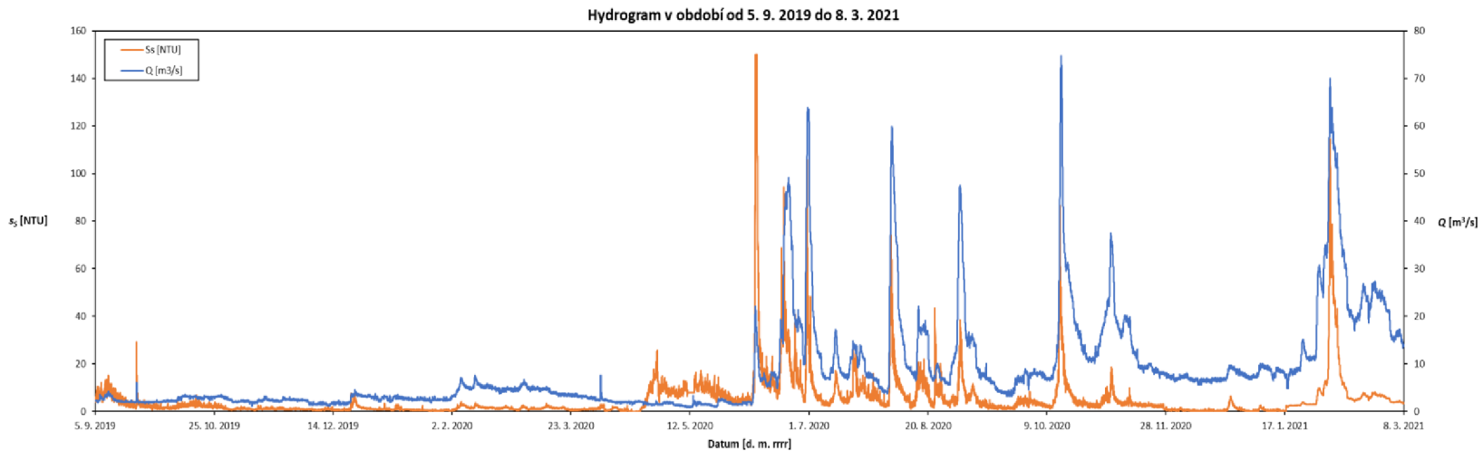
Obr. 45. Hydrogram vzniklý metodou korekce dat pomocí vyhlazení a doplnění, vodoměrný profil Příbice
