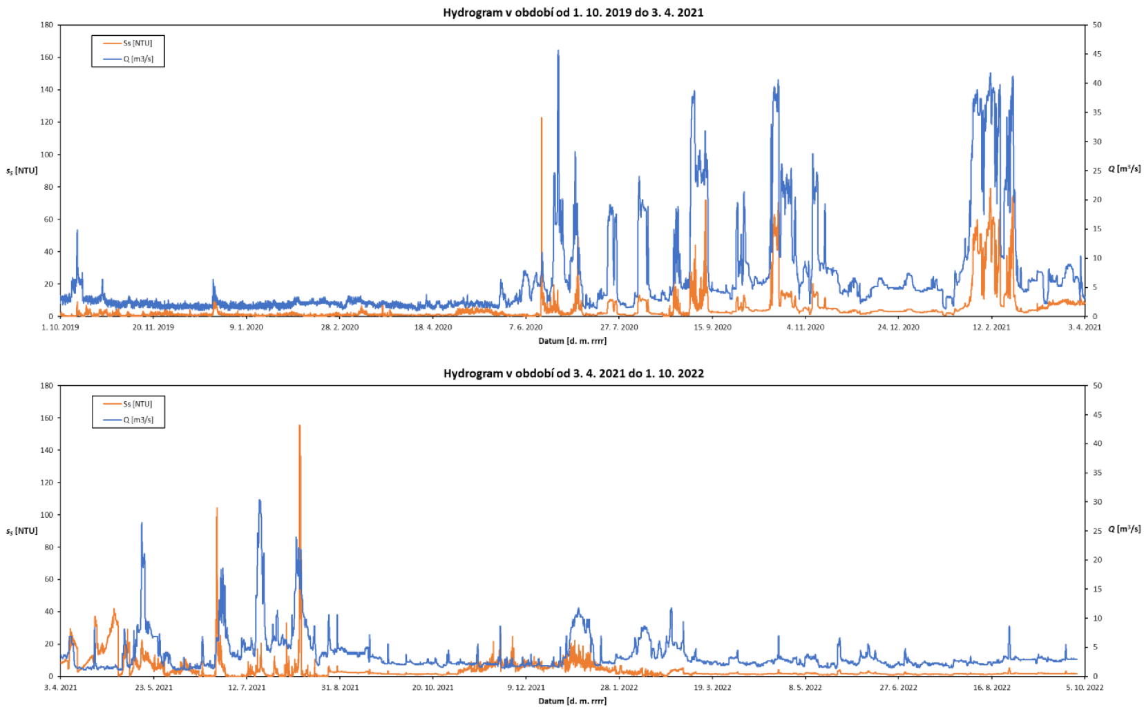
Obr. 32. Hydrogram vzniklý metodou korekce dat pomocí vyhlazení a doplnění vodoměrný profil Hevlín
