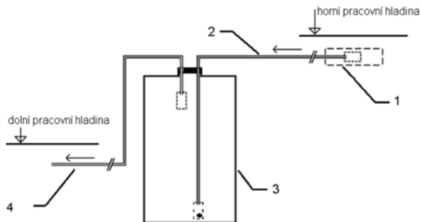
Obr. 7. Schéma detritového kontinuální vzorkovače: 1 – sací koš umístěný do vodního toku, 2 – přívodní flexibilní potrubí, 3 – tělo se sedimentačním prostorem, 4 – odtokové flexibilní potrubí; horní hladina znázorňuje místo uložení sacího koše ve výše položené části toku a dolní hladina znázorňuje ústí odpadního potrubí v níže položené části toku s velkým spádem [7]
