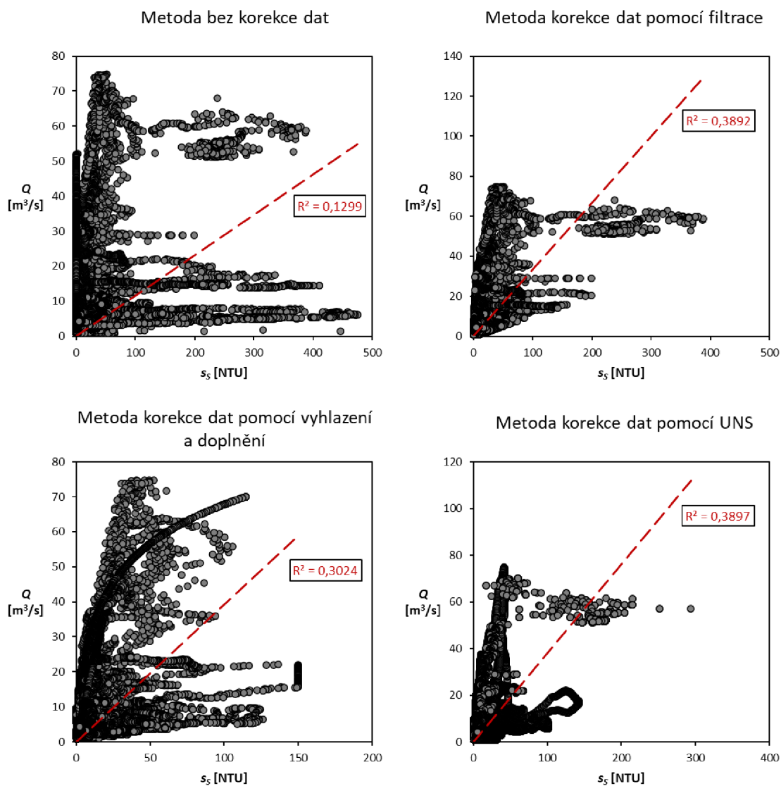
Obr. 48. Analýza úspěšnosti korekce dat ve vodoměrném profilu Příbice
