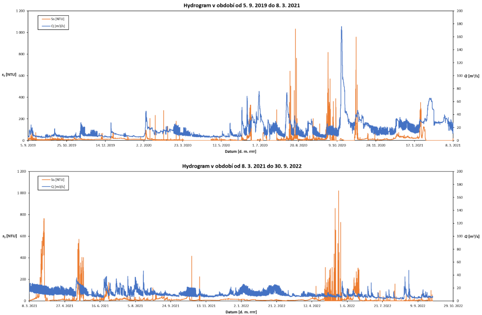
Obr. 51. Hydrogram vzniklý metodou bez korekce dat, vodoměrný profil Židlochovice
