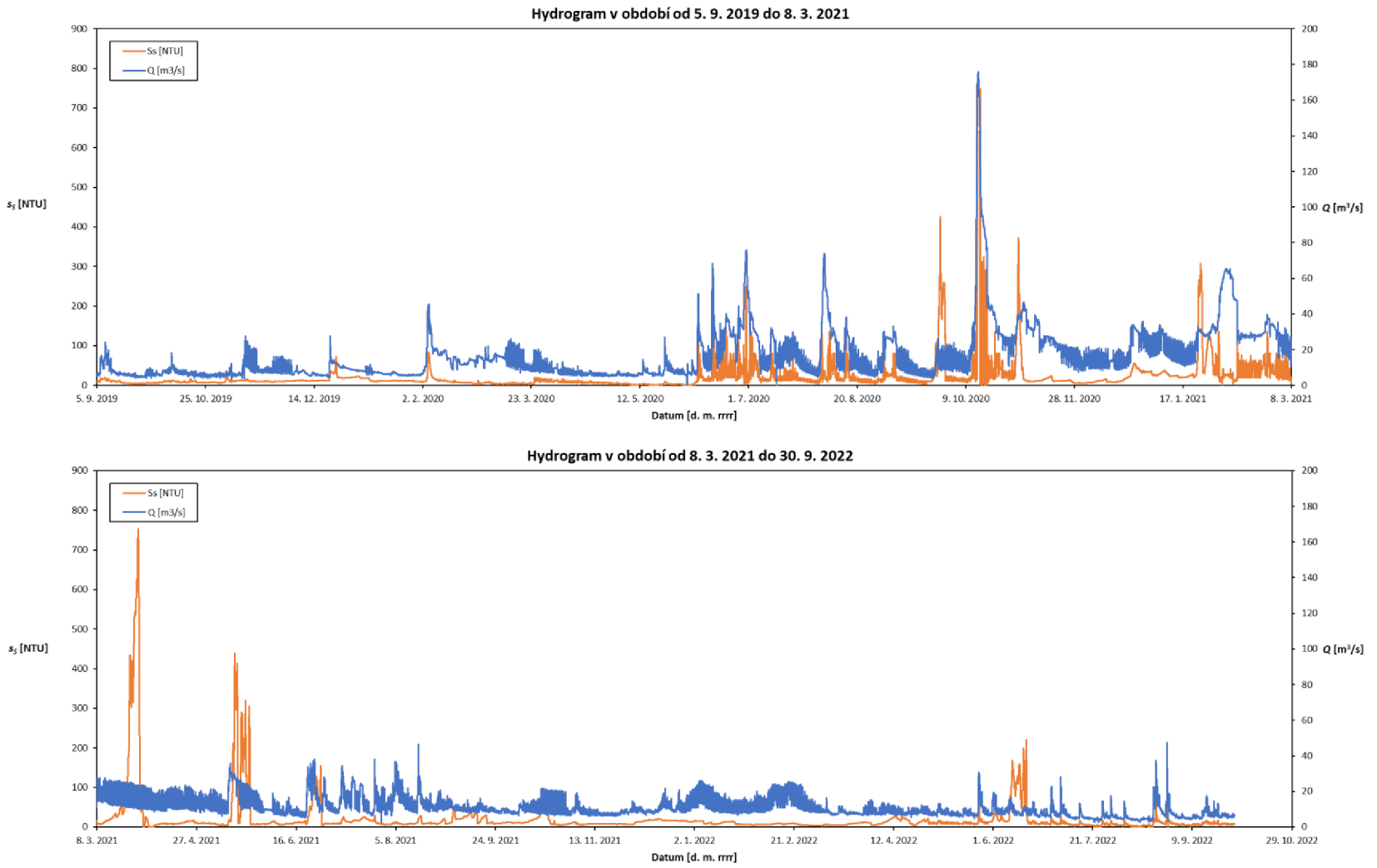
Obr. 56. Hydrogram vzniklý metodou korekce dat pomocí UNS, vodoměrný profil Židlochovice
