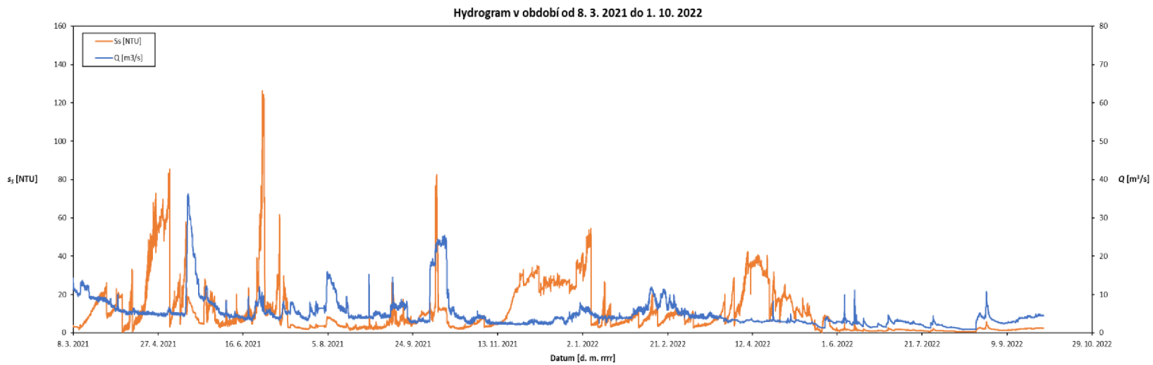
Obr. 45. Hydrogram vzniklý metodou korekce dat pomocí vyhlazení a doplnění, vodoměrný profil Příbice
