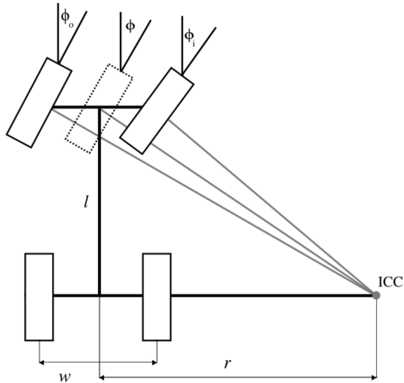
Obrázek 3.9: Ackermannovo řízení [20]
