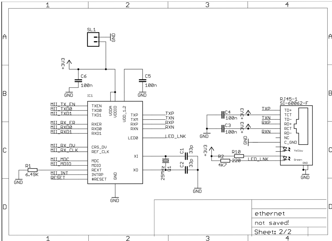
Obr. A.2: Schéma zapojení vývojového modulu pro ethernet, list 2
