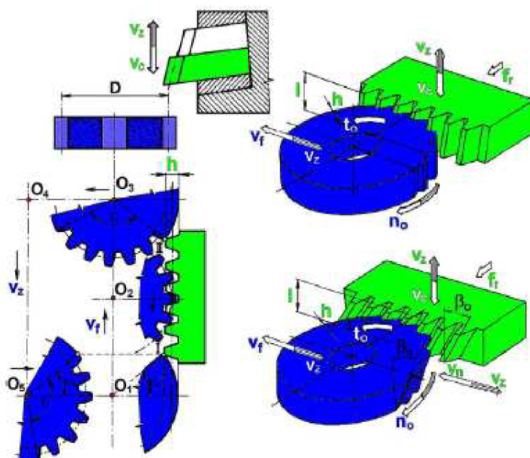
Obr.1.5 Obrážení hřebenovým nožem [5]
