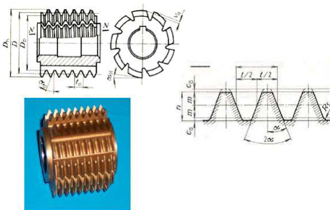
Obr.2.3 Odvalovací fréza [7] [8]
