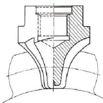
Obr.2.1 Čepová fréza [5]
