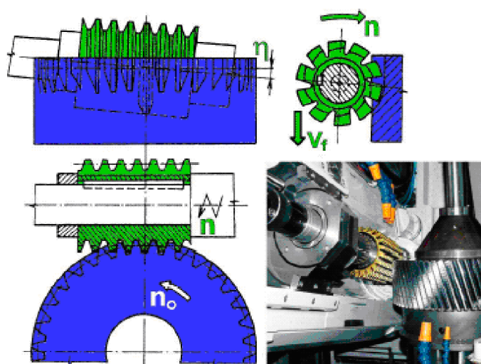
Obr.1.4 odvalovací frézování přímého ozubení [5]
