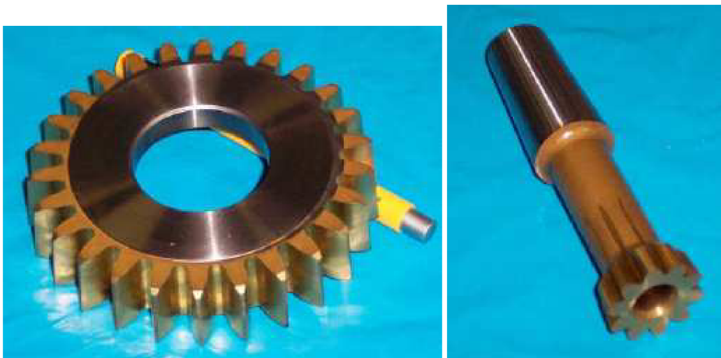
Obr.2.6 Obrážecí kotoučový nůž, obrážecí kotoučový nůž stopkový [8]
