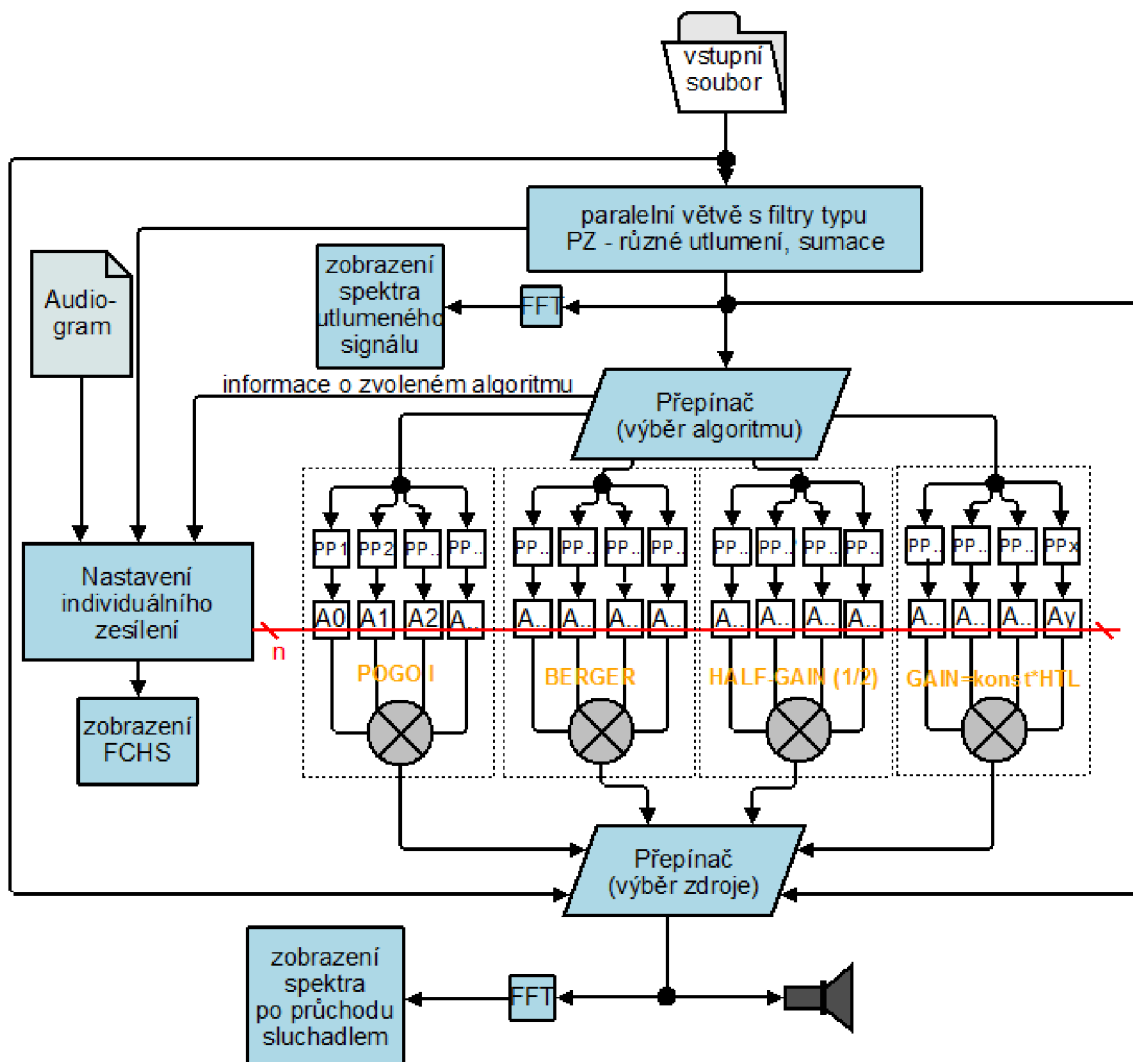
Obr. 6.1: Blokové schéma sluchadla
