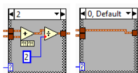
Obr. 6.10: Struktura úpravy stereozvuku (vlevo) a průchod pro monozvuk (vpravo)
