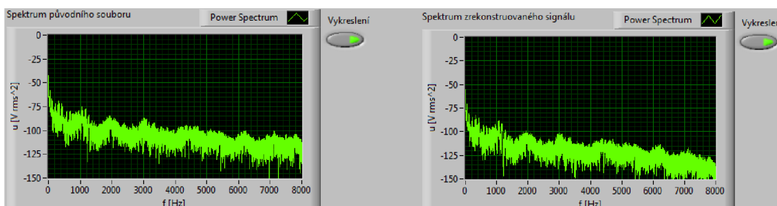
Obr. 6.28: Spektrum signálu na vstupu a po průchodu sluchadlem
