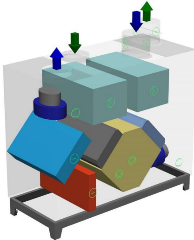
Obrázek 38 Axonometrie VZT jednotky č. 3
