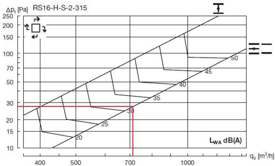
Obrázek 21 Určení tlakové ztráty vířivé vyústí RS16 dimenze 315
