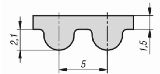
Obrázek 14 Ozubený řemen HTD 5M [9]
