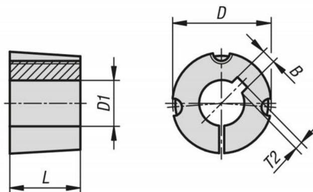
Obrázek 11 Kuželové upínací pouzdro [7]
