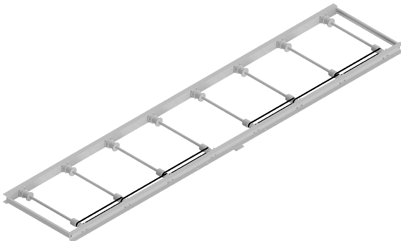
Obrázek 5 Konstrukce zdvižného stolu
