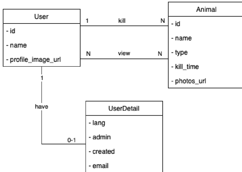
Obr. 6.7: Výsledný doménový model lokálnej databázy
