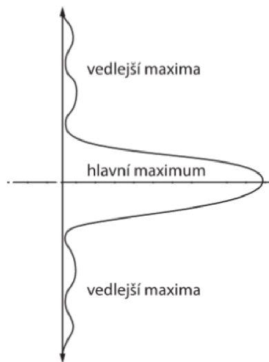
Obrázek 2.3: Difrakční obrazec. [8]
