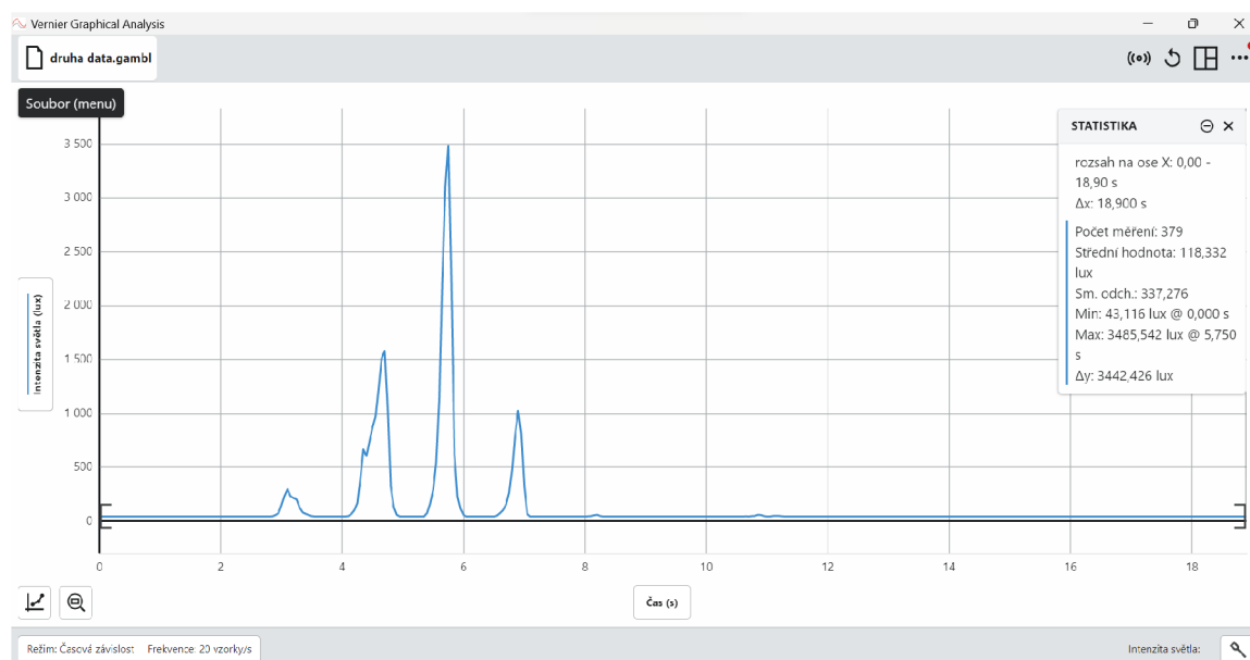
Obrázek 4.7: Difrakční obrazec.
