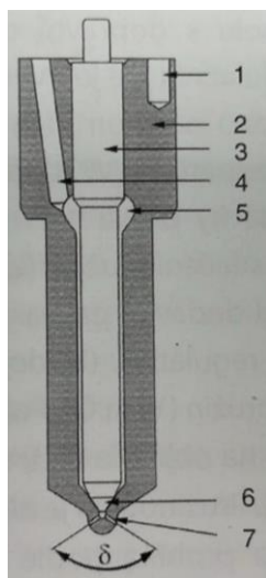
Obr. 18 – Vstřikovací tryska otvorová (HROMÁDKO, a další, 2011)
