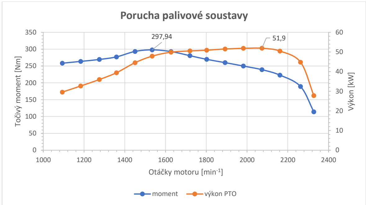
Graf 3 – Vnější otáčková charakteristika motoru s poruchou palivové soustavy
