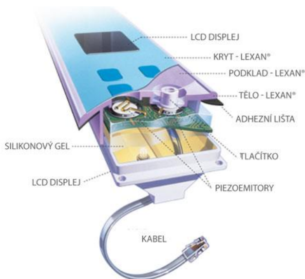
obr. 2-17 Ovládací panel vířivky R6L [25]
