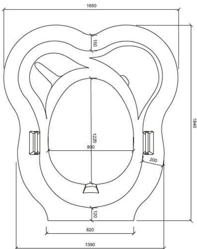
obr. 2-19 Rozměry produktu Active Birth Pool v milimetrech. [10]
