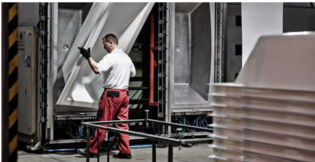
obr. 2-20 Výroba van Ravak [31]
