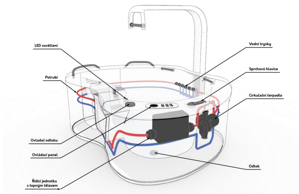
obr. 6-2 Uspořádání vnitřních komponent
