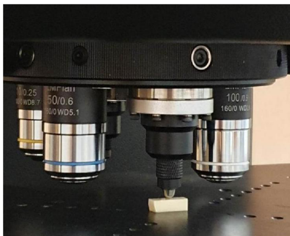
Obr. 18 Otáčecí věž s indentory a objektivy
