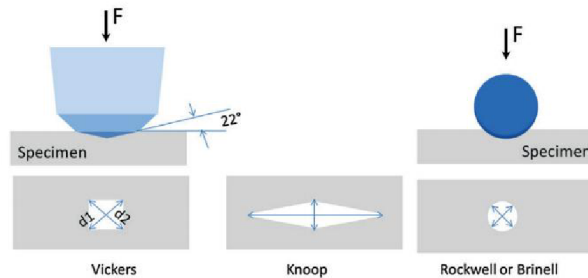
Obr. 5 Otisky indentoru pro jednotlivé zkoušky tvrdosti (16)
