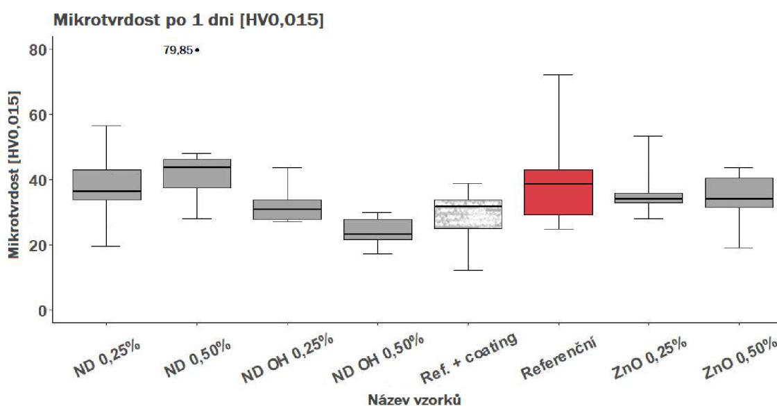
Graf 8: Mikrotvrdość po 1 dni
