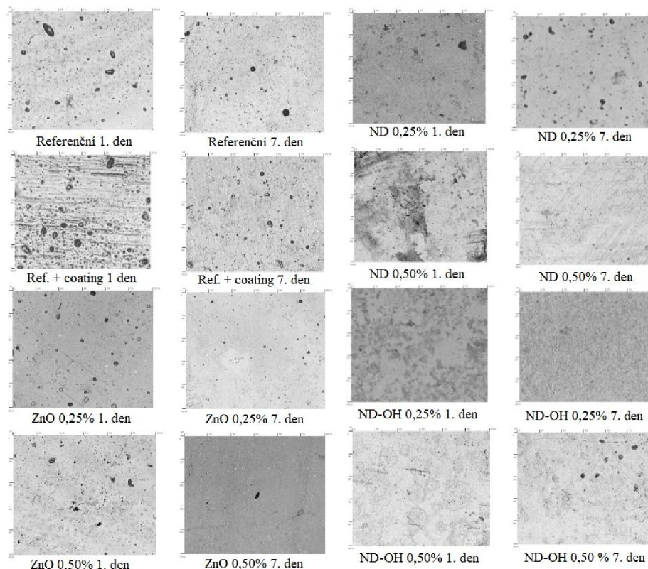
Obr. 22 Povrchová poréznost (tmavé oblasti v obrazech jsou znázorněním pórů)
