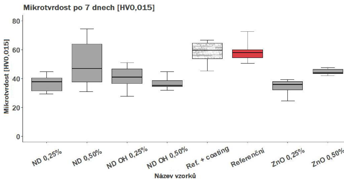
Graf 9: Mikrotvrдость po 7 dnech
