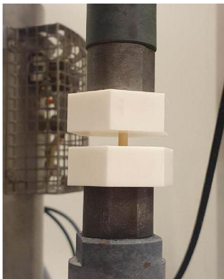
Obr. 16 Umístění vzorku mezi dva pravidelné šestiboké hranoly
