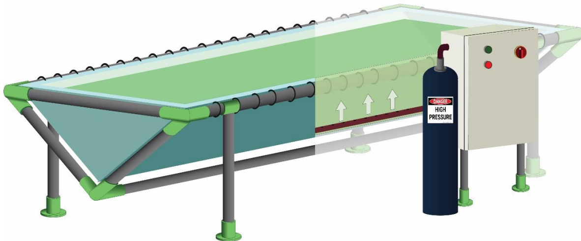
Obr. 5: Moderný race-way pond, pohyb média zabezpečuje aerácie pomocou hadičku umiestnenej na dne nádrže, nadrž sa aeruje pomocou neupraveného vzduchu alebo obohateného o \text{CO}_2 , modifikované podľa Zuckermann et al. 2015.
