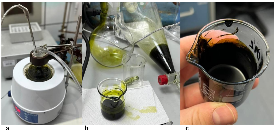
Obr. 38: Odparovanie chloroformu a: odparovanie organického rozpušťača chloroformu zahrievaným vo variči a odvetraný plynným dusikom; b: posledných 20 ml zmesi, ktoré odparoval na indukčnom variči; c: finálne surové lipidy.
