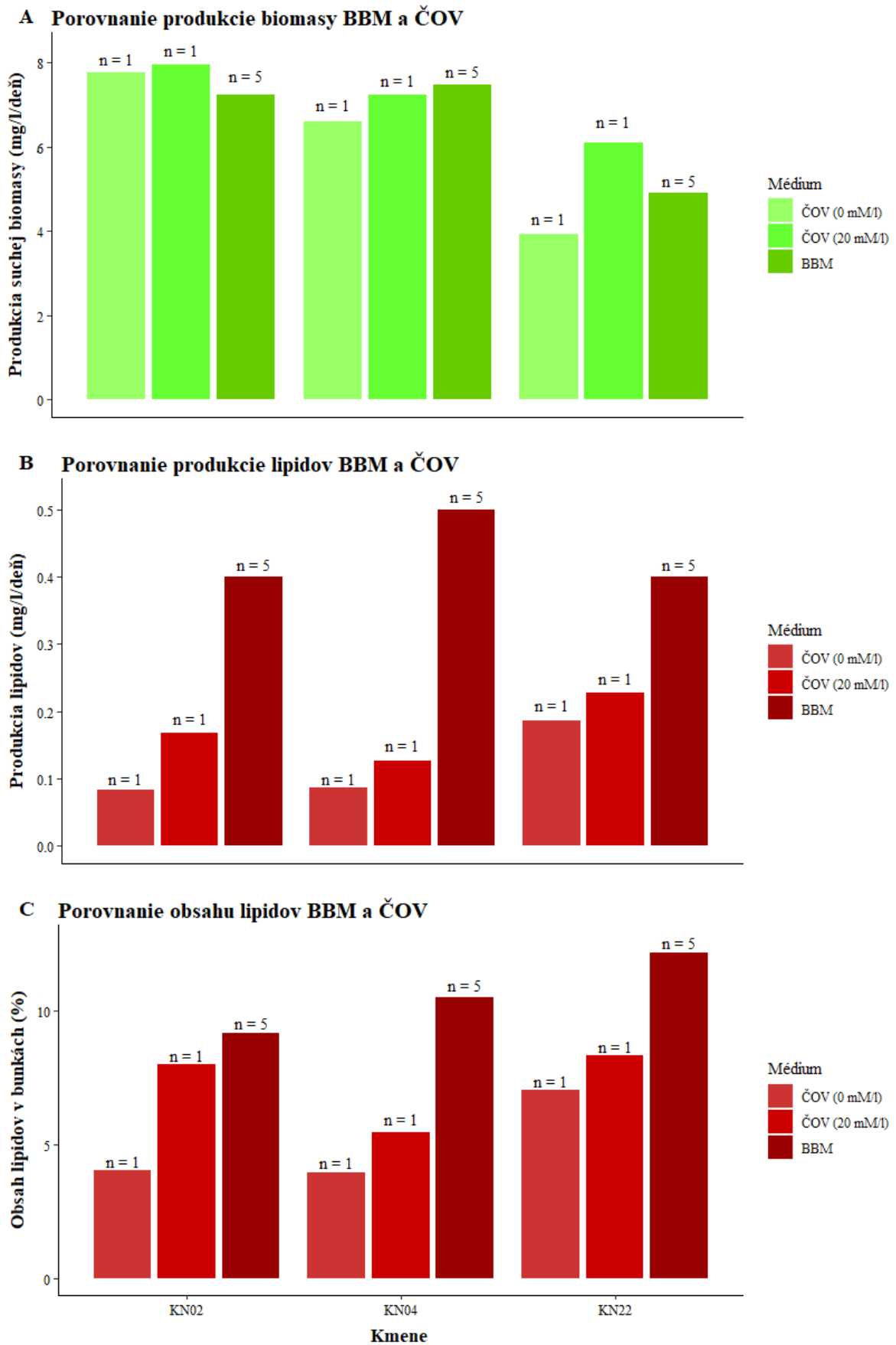
Obr. 20: Finálna produkcia média BBM a vody z ČOV, čísla nad stĺpcami znázorňujú počet sledovanie v jednotlivých mediach.
