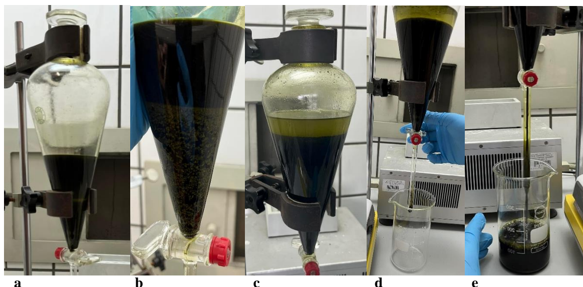
Obr. 37: Extrakcia lipidov pomocou zmesi chloroform – metanol; a: rozrušenie buniek pomocou metanolu; b: pridanie chloroformu; c: pridanie roztoku 0,9% NaCl a vytvorenie bifázického rozdelenia; d,e: odstraňovanie dolnej vrstvy s chloroformom a lipidmi.
