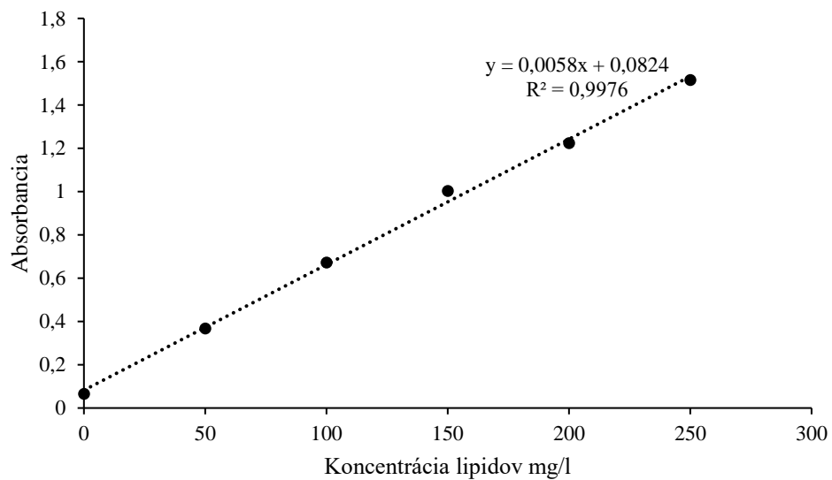
Kalibračná krivka váhy lipidov
