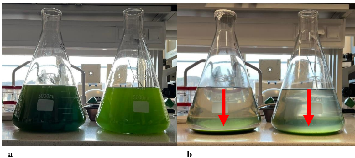
Obr. 34: Sedimentácia (sedimentácia biomasy za 16 hodín)
