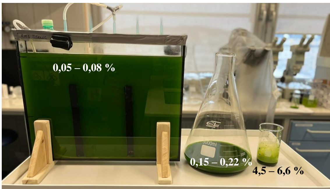
Obr. 35: Objemový pomer medzi biomasou pred a po zakoncortovaní; % znázorňujú množstvo gramov na liter, reaktor predstavuje nezakoncortovanú biomasu, v banke je zakoncortovaná biomasa po sedimentácií 4 litrov média, v kadičke je vysedimentovaná biomasa z banky po zakoncortovaná centrifugácií.
