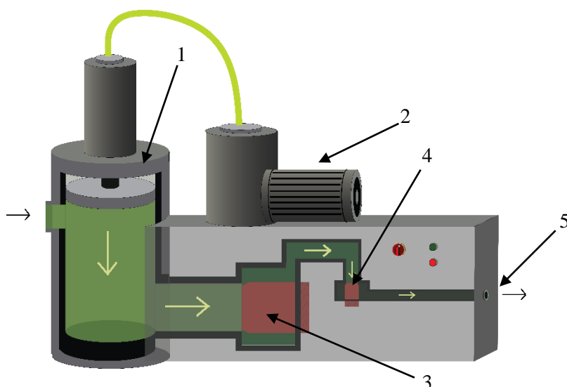
Obr. 8: Vysokotlakový lis na rozrúšanie buniek v biomase 1 – piest; 2 – hydraulický motor; 3 – primárny nastavovateľný lisovací zub; 4 – sekundárny zub; 5 – zlisovaná biomasa (modifikované z www.homogenizers.net ).
