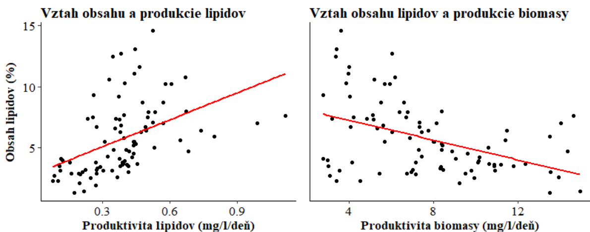
Obr. 17: Vzťah medzi obsahom lipidov a dennou produkciou lipidov a biomasy; červená čiara predstavuje trendovú spojnicu.
