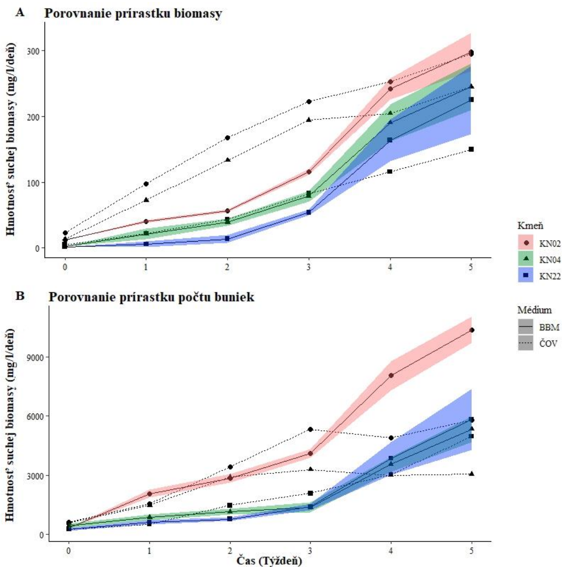
Obr. 19: Produkcia v laboratórnom médiu BBM a vo vodou z ČOV, farebné pole okolo kriviek s médiom BBM znázorňuje štandardnú odchýlku; BBM n = 5, ČOV n = 1; kvôli malého množstvu vody z ČOV som nemohol uskutočniť opakovania.
