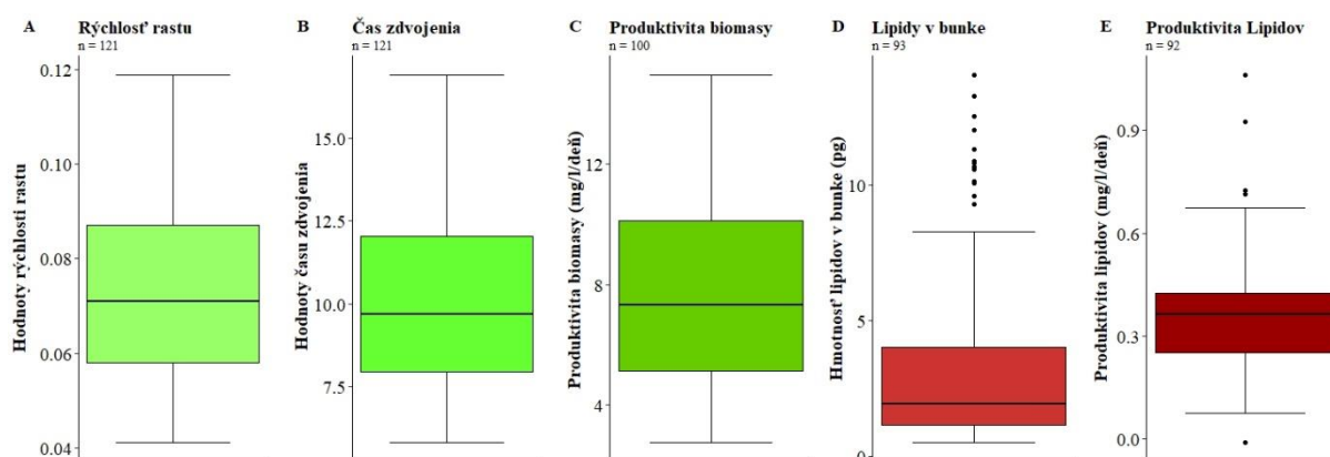
Obr. 15: Prehľad celkovej produkcie a efektivity riasy Scenedesmus sp.; písmená A až E znázorňujú jednotlivé parametre, viac informácií pozri nižšie.
