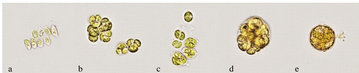
Obr. 23: Efekt salinity na morfológiu buniek; a – 0 mM/l; b – 85,5 mM/l; c – 171 mM/l; d – 256,5 mM/l; e – 342 mM/l.
