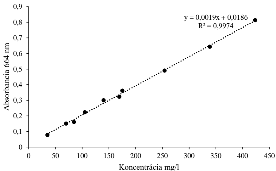
Kalibračná krivka suchej váhy biomasy
