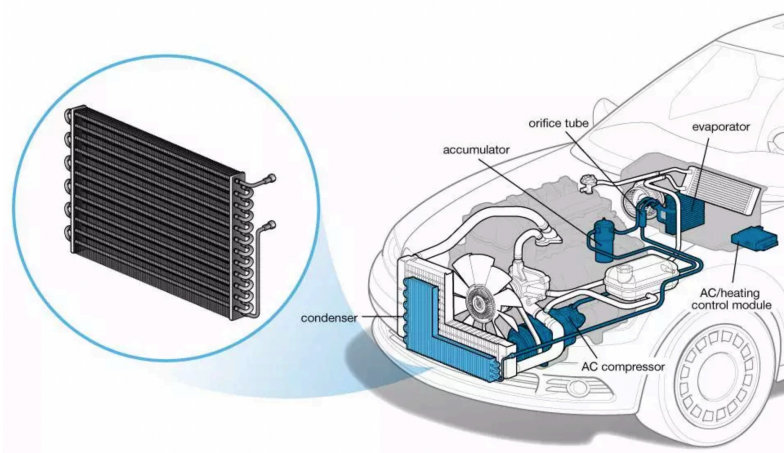
Obrázek 13: Ilustrace kondenzátoru
