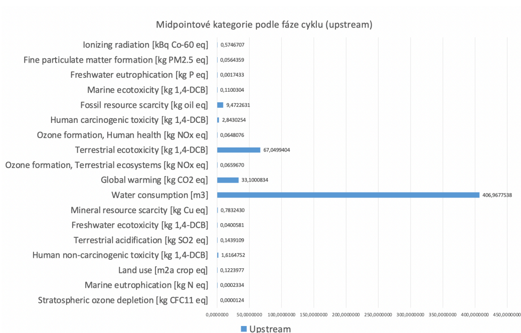
Obrázek 25: Midpointové kategorie dopadů dle fáze cyklu (upstream) Zdroj: vlastní výstup
