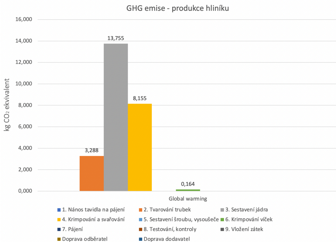
Obrázek 22: GHG emise - produkce hliníku Zdroj: vlastní výstup
