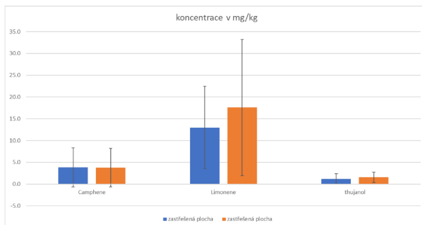
Obrázek č. 9: Graf vybraných sloučení po aplikaci rovnice externí kalibrační křivky (Chybové úsečky jsou \pm 1xSD )
