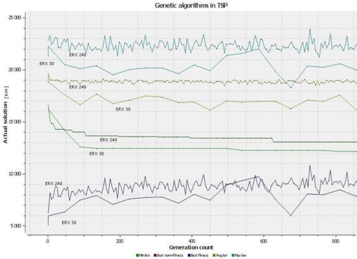
Obrázek 3.17 Průběh křížní ERX s 30 a 240 jedinci
