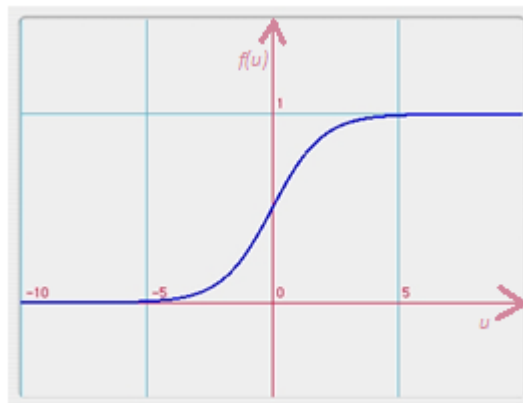
Obrázek 3.36 Sigmoida
