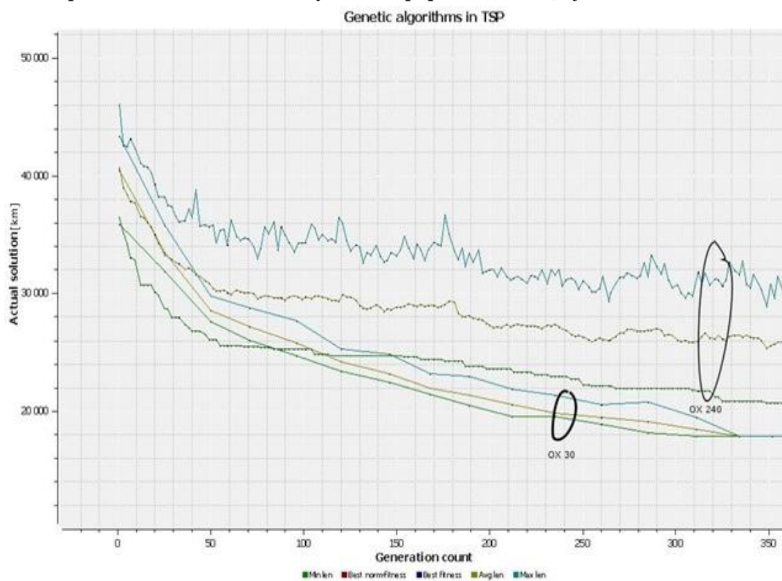
Obrázek 3.19 Průběh křížení OX s 30 a 240 jedinci
