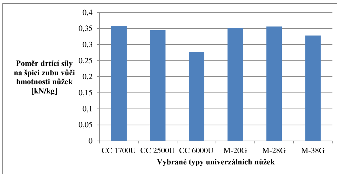
Obr. 13 Graf poměru drtící síly na špičce zubu ku hmotnosti nůžek
