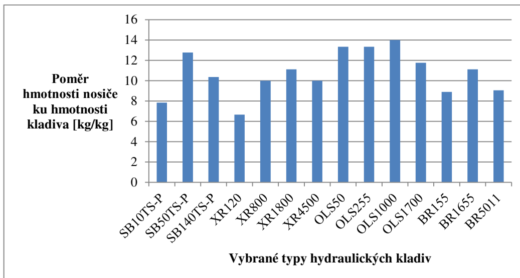
Obr. 5 Graf poměru minimální hmotnosti nosiče vůči hmotnosti hydraulického kladiva
