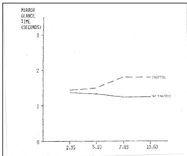
Obr. 36: Vliv šířky zrcátka na délku pohledu [40]
