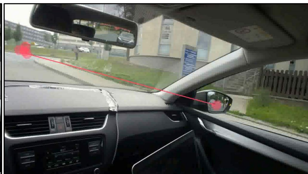
Obr. 52: Počátek fixace [75]
