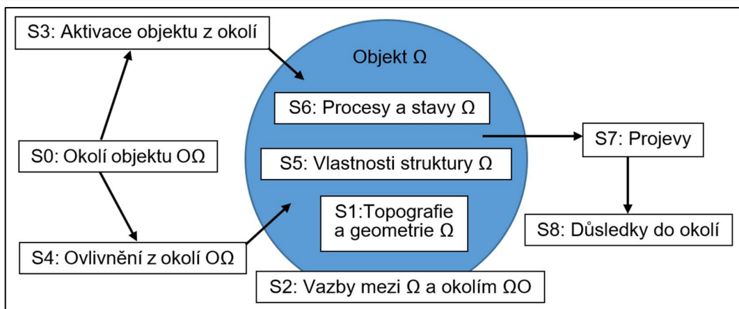
Obr. 38: Systém veličin [4]
