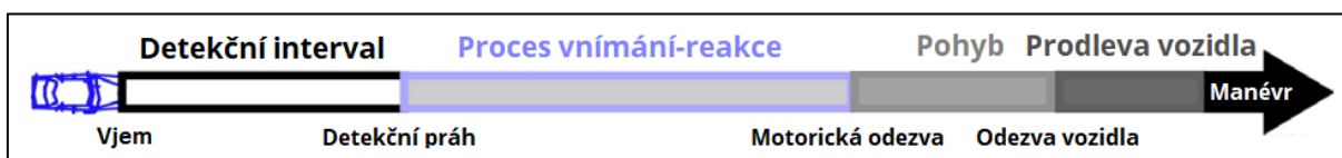
Obr. 19: Složky reakční doby dle Muttarta [23](úprava autor)
