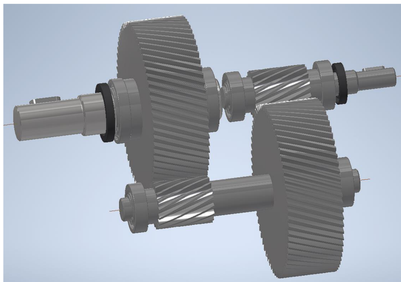
Obr. 7 Ozubené soukolí
