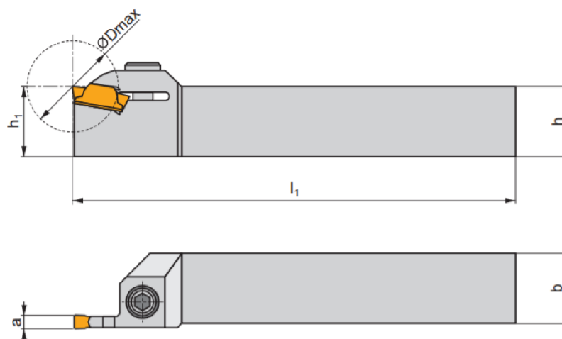
Obr. 29 Vnější zapichovací nůž [13].
