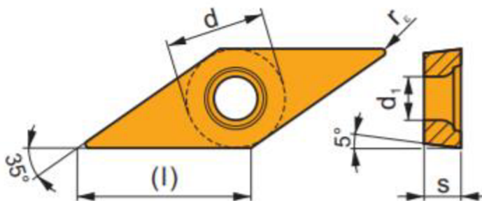
Obr. 26 Dokončovací VBD [13].
