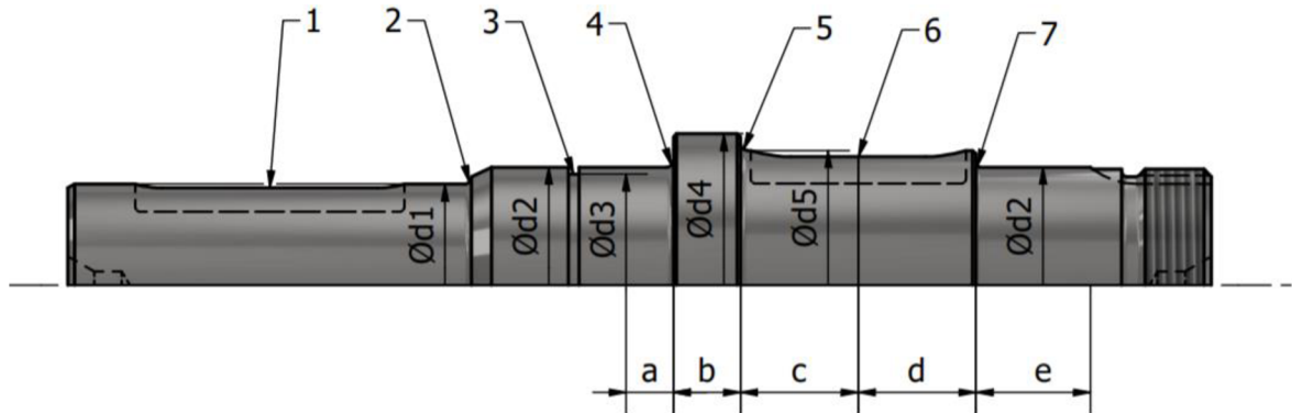
Obr. 12 Kontrolovaná místa na výstupním hřídeli
