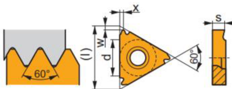
Obr. 28 Závitová VBD [13].
