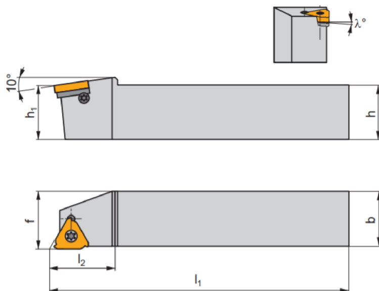
Obr. 27 Vnější závitový nůž [13].
