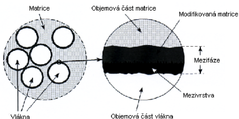
Obr. 6: Schématické znázornění kompozitní mezifáze.[8]
