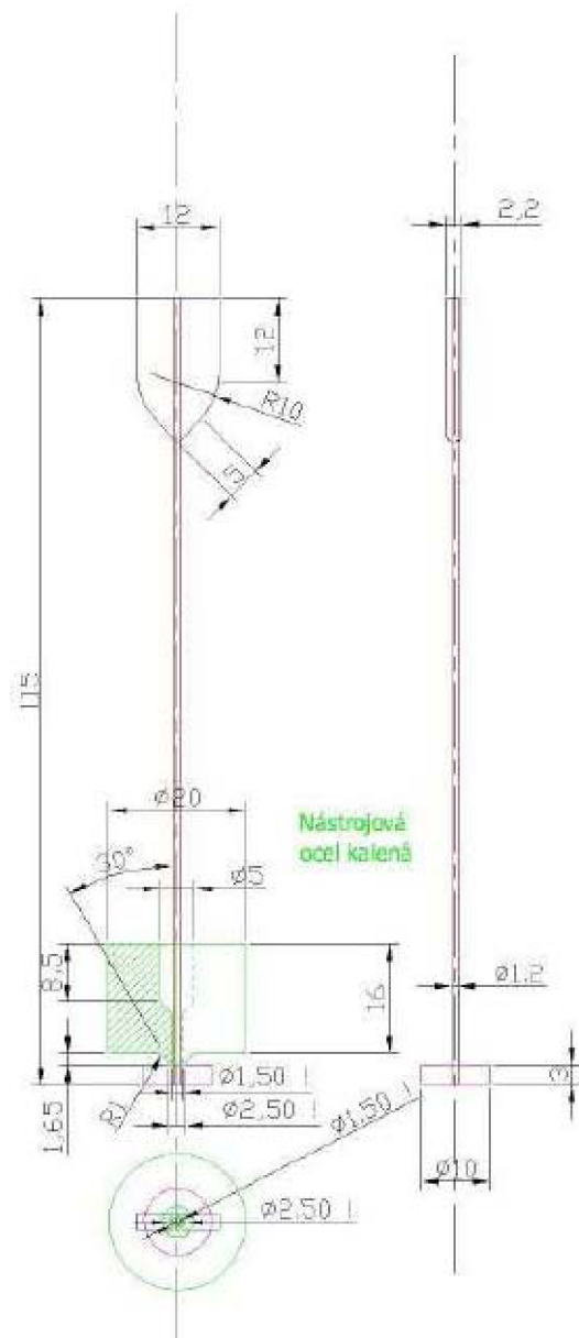
Obr. 12: Schéma vzorku kompozitu
