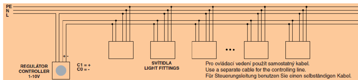
Obrázek 6: Zapojení analogového regulátoru [1]
