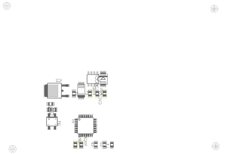
Obrázek 31: Rozmístění součástek EP strana BOTTOM
