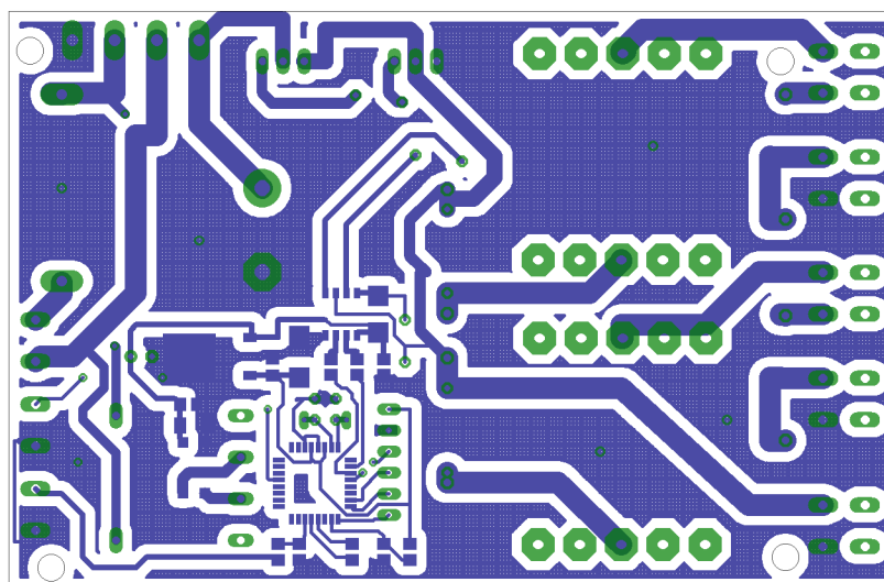
Obrázek 34: DPS EP ze strany BOTTOM
