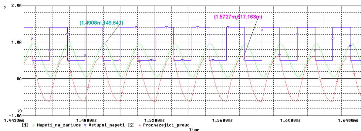
Obrázek 22: Průběh napětí a proudů při provozu zářivky
