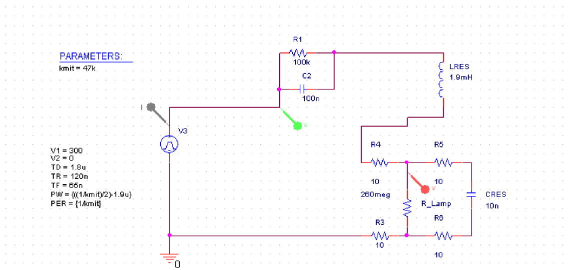
Obrázek 18: Náhradní schema zapojení modelu zářivky
