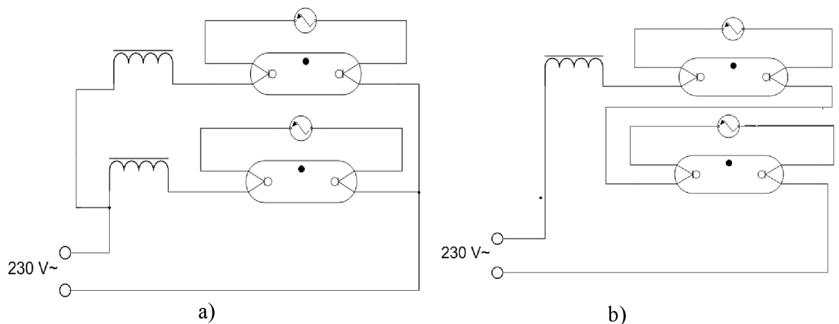
Obrázek 2: Řazení trubic: a) paralelní b) sériové
