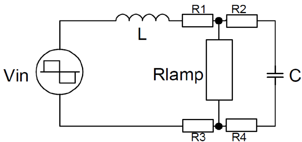
Obrázek 4: Náhradní schema zapojení zářivky [9]
