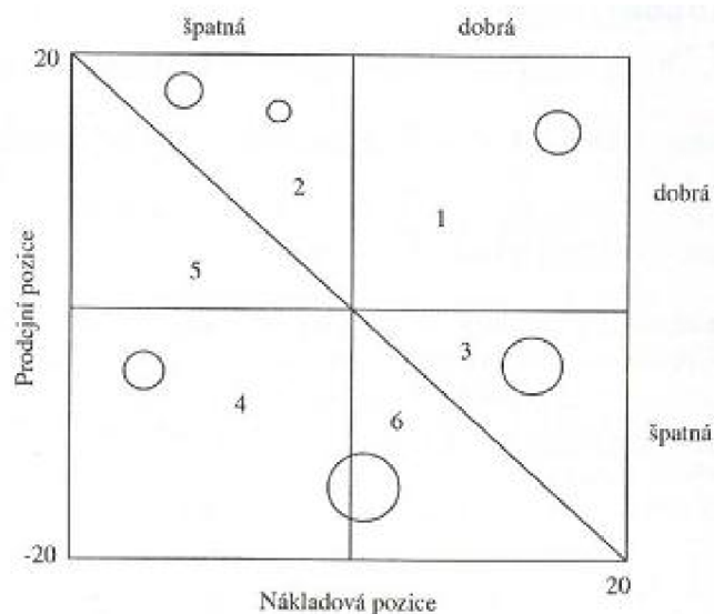
Obr. 19 Matice přežití[9]
