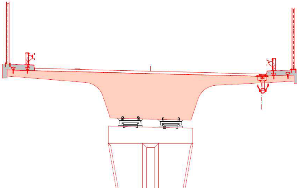
Obrázek 3 - Jednotrámová varianta
