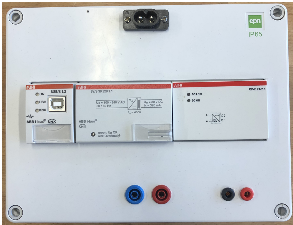
Obrázek 5.4: Modul 230 VAC, 2. typ
