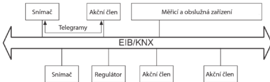
Obrázek 3.1: Komunikace KNX/EIB [3]
