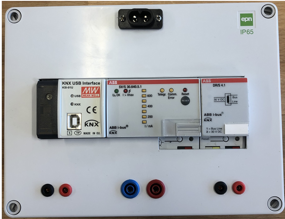
Obrázek 5.3: Modul 230 VAC, 1. typ
