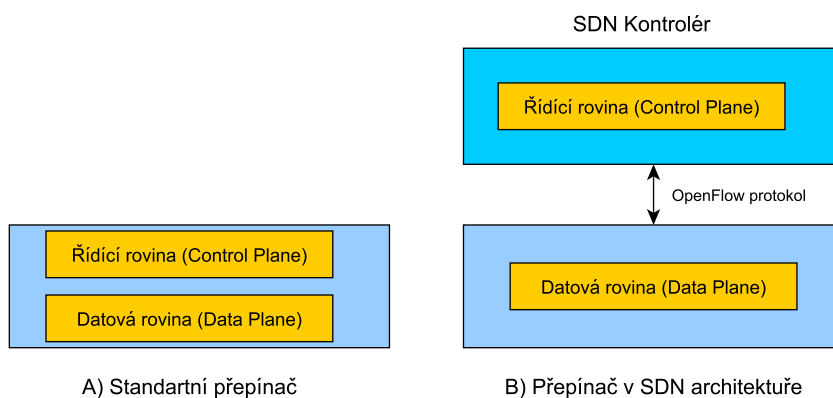
Obr. 4.1: Srovnání přepínačů
