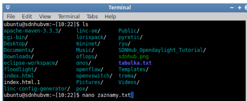
Obr. 4.27: Terminálové okno
