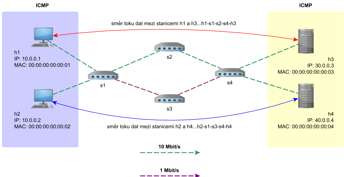
Obr. 4.46: Schéma topologie pro samostatný úkol
