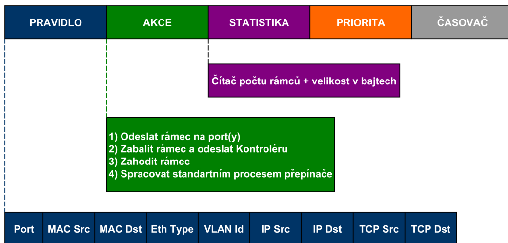
Obr. 2.1: Struktura OpenFlow tabulky
