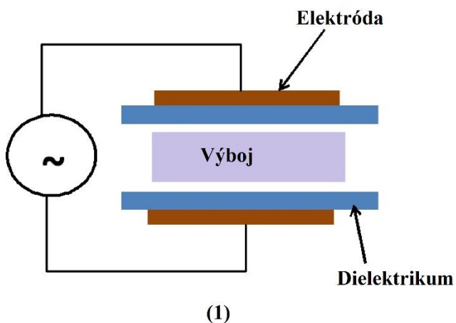
Obrázok 7: Schematické znázornenie dielektrického bariérového výboja (1) a dielektrický bariérový výboj v praxi (2) [21]
